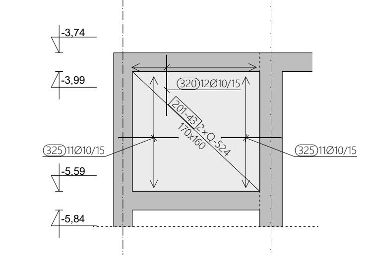
ARMATURA ZIDA IZMEĐU OSI 3.07 I 3.08, M 1:50
