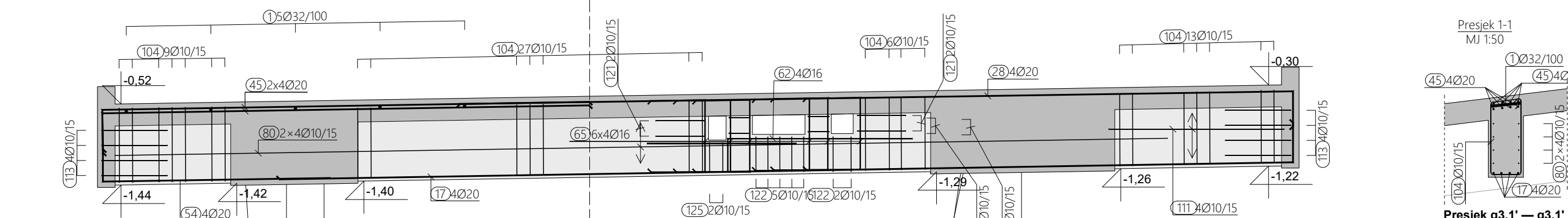
ARMATURA GREDE 3.2, M 1:50
