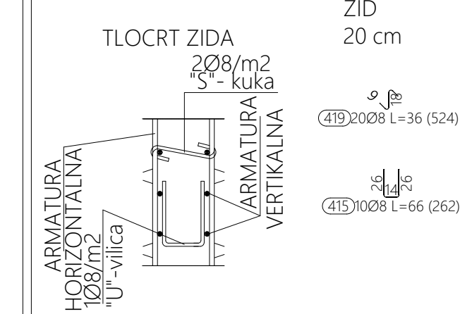
DETALJ POSTAVLJANJA DISTANCERA U ZID E-2
