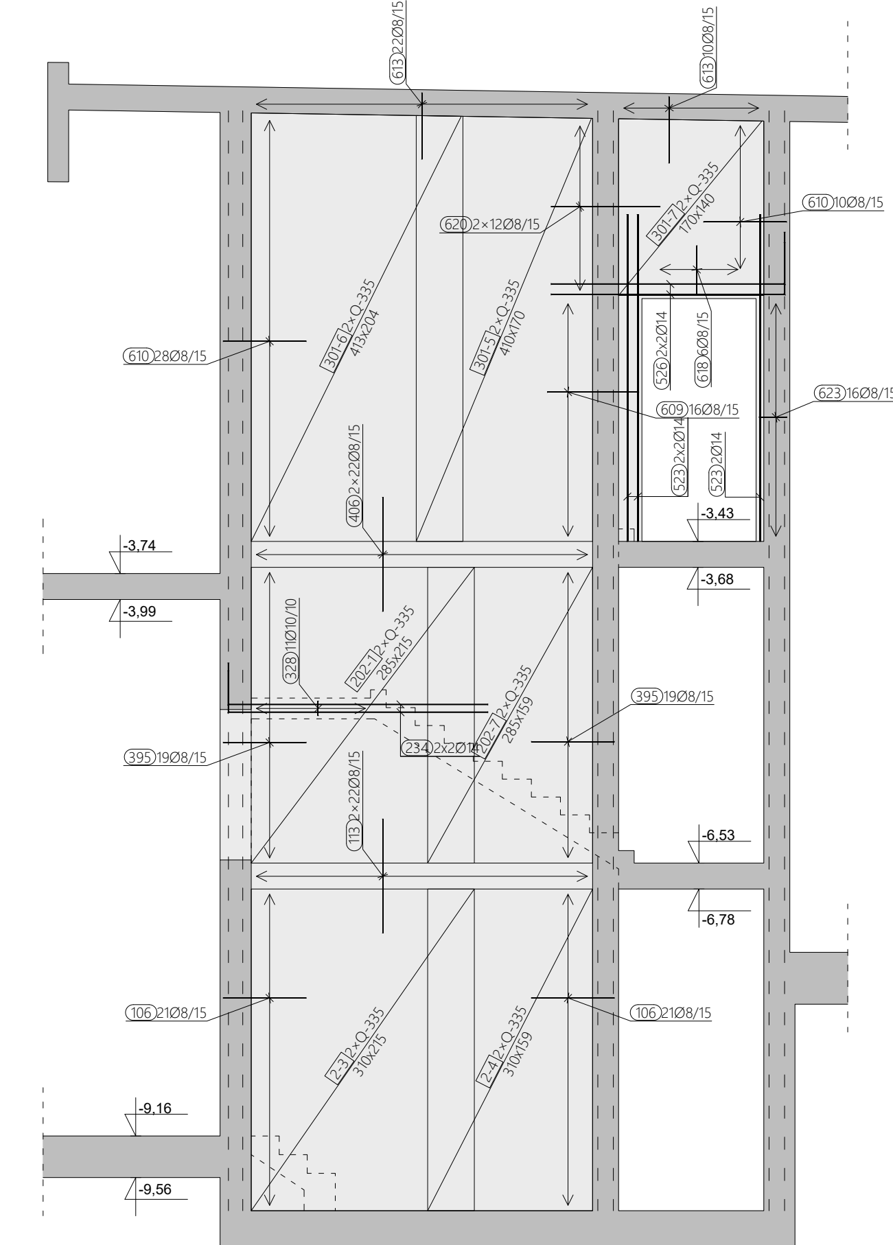
ARMATURA ZIDA U OSI 3.11, M 1:50
