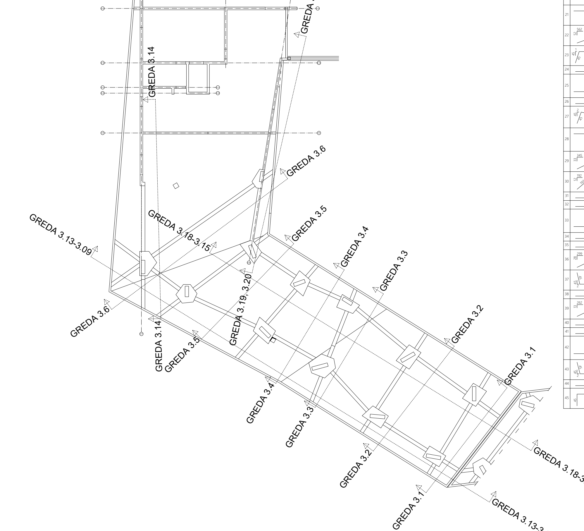
DISPOZICIJA GREDA
