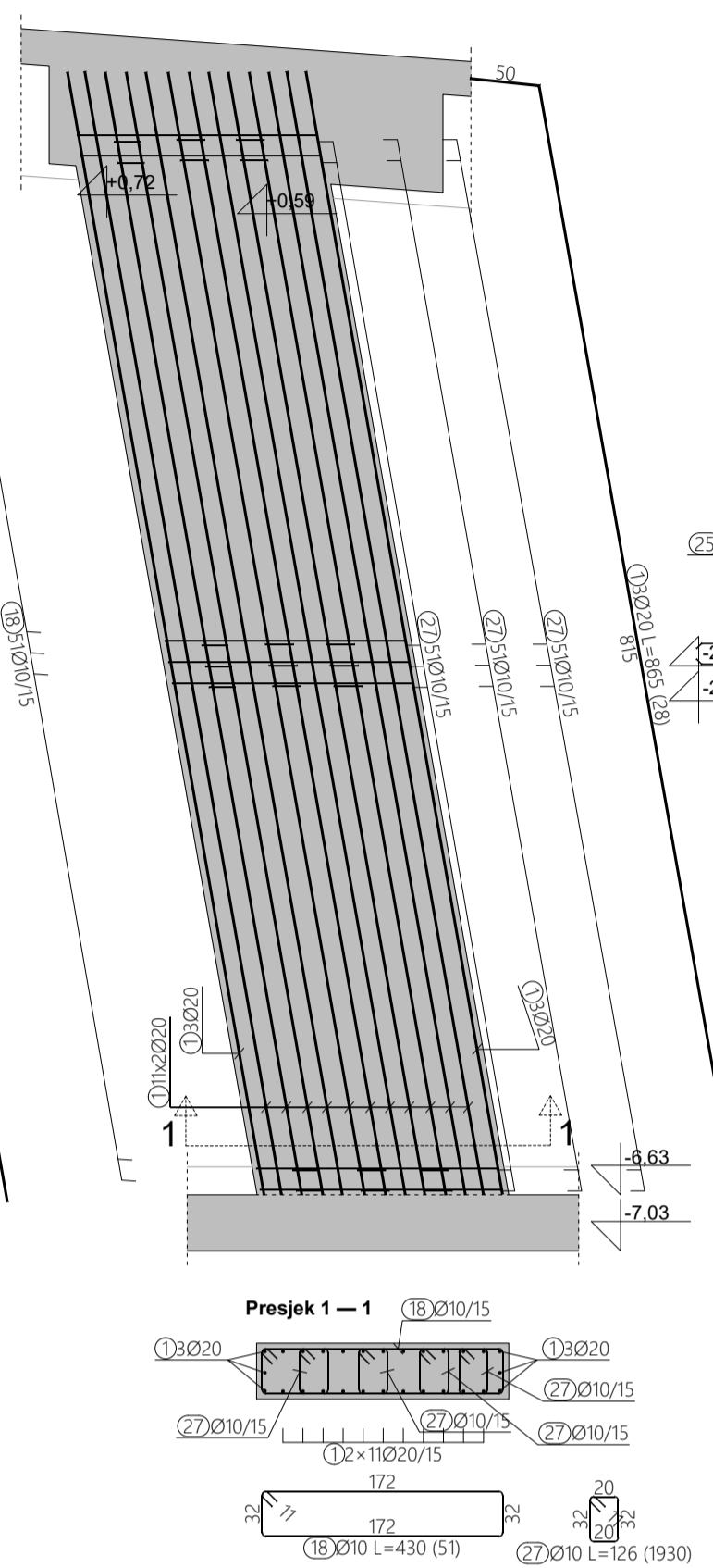
ARMATURA STUPA 3.12, M 1:50
