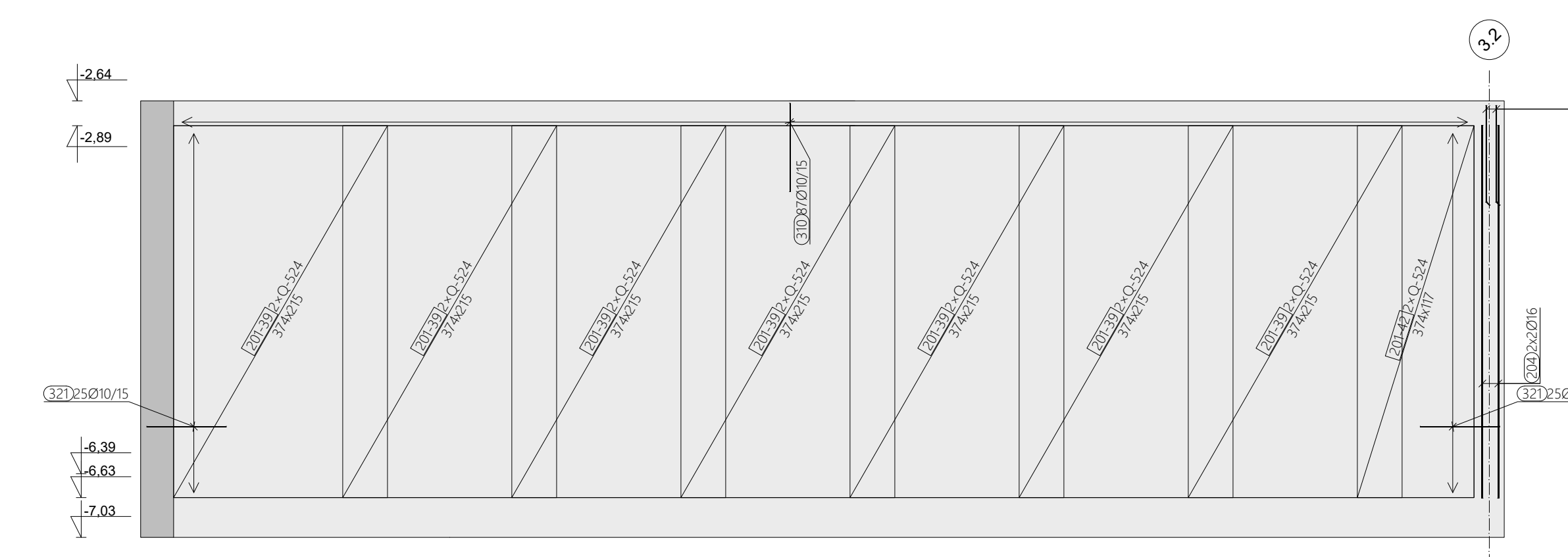
ARMATURA ZIDA U OSI 3.3, M 1:50
