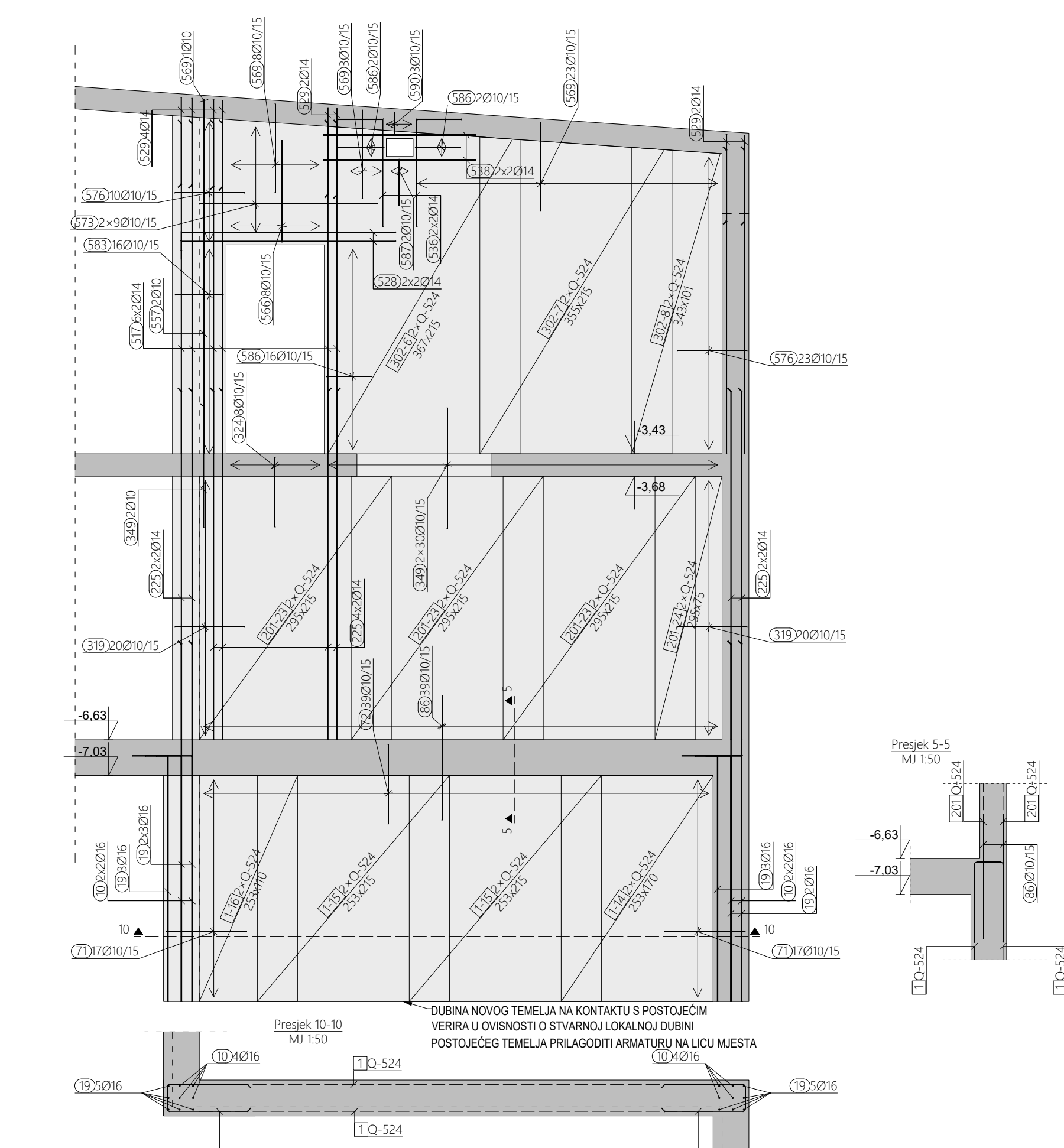
ARMATURA ZIDA U OSI 3.25, M 1:50
