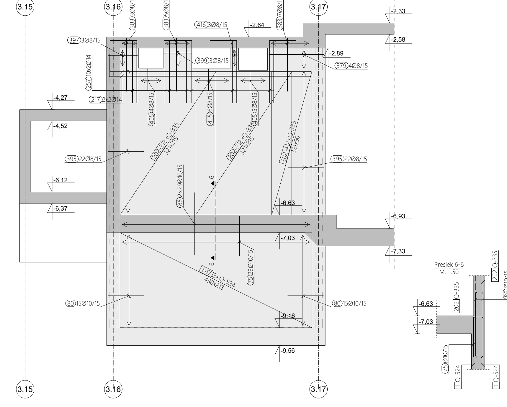
ARMATURA ZIDA U OSI 3.7, M 1:50
