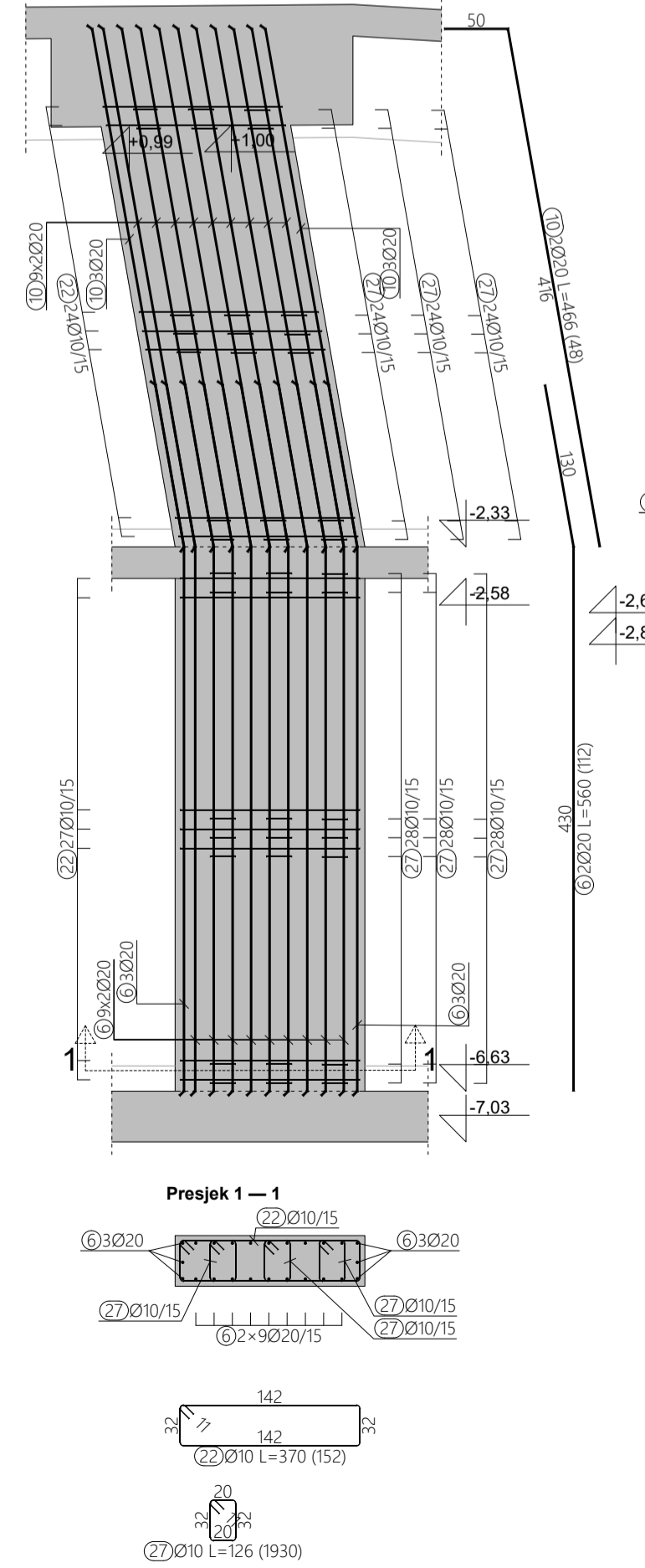
ARMATURA STUPA 3.10, M 1:50
