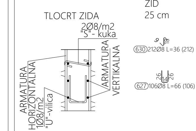
DETALJ POSTAVLJANJA DISTANCERA U ZID E-1
