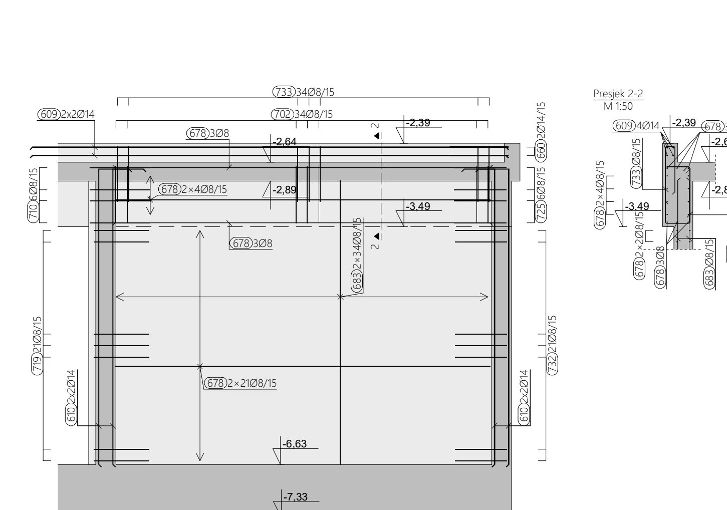
ARMATURA ZIDA U OSI 3.27 M 1:50
