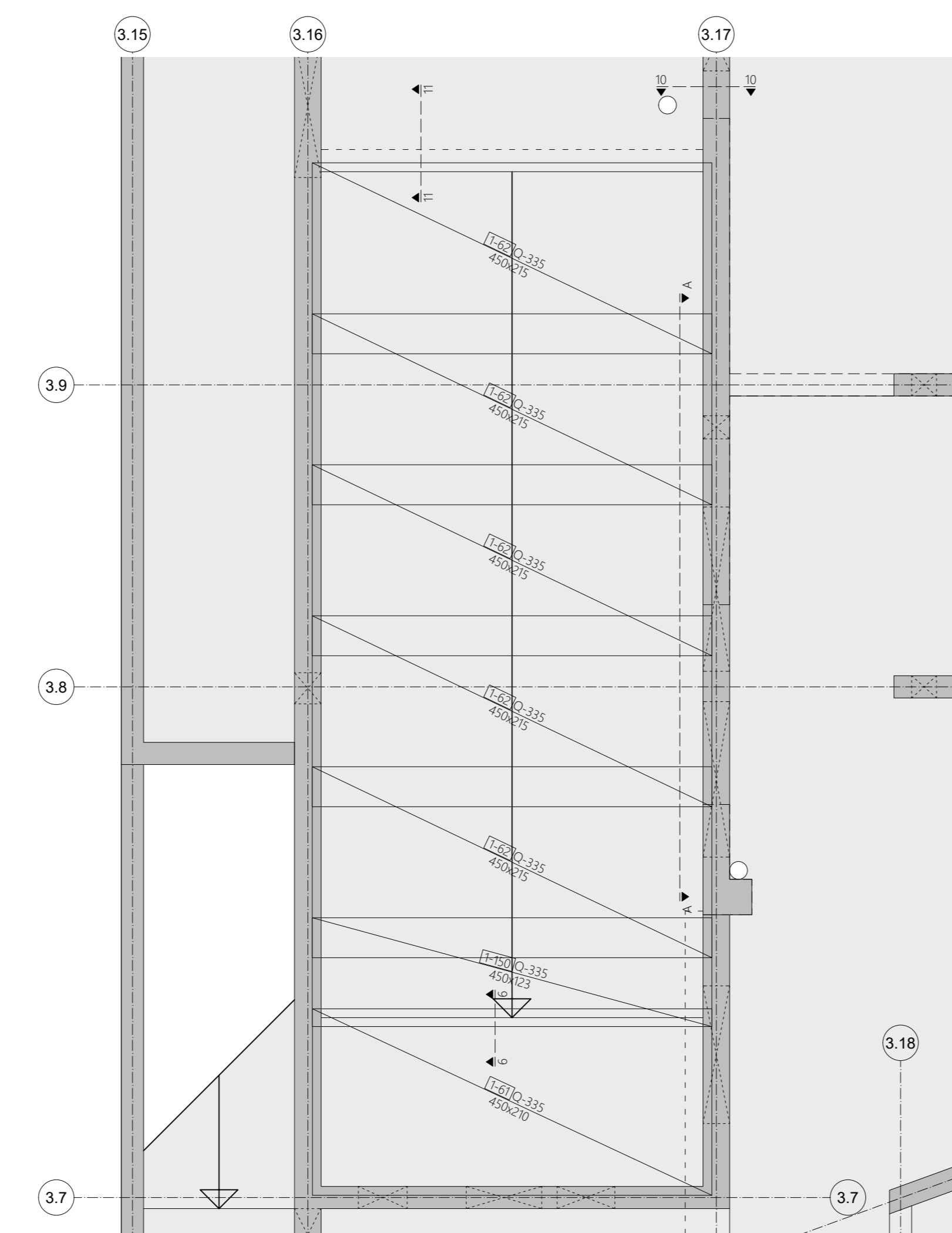
ARMATURA GORNJE ZONE, PLOČA NA VISINI -3.33 do -2.64/-2.89, M 1:50
