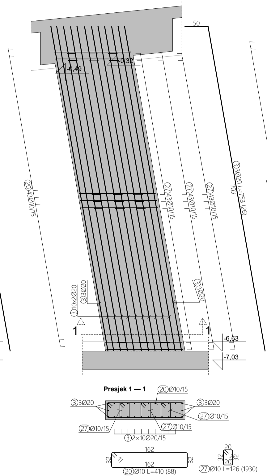
ARMATURA STUPA 3.3, M 1:50
