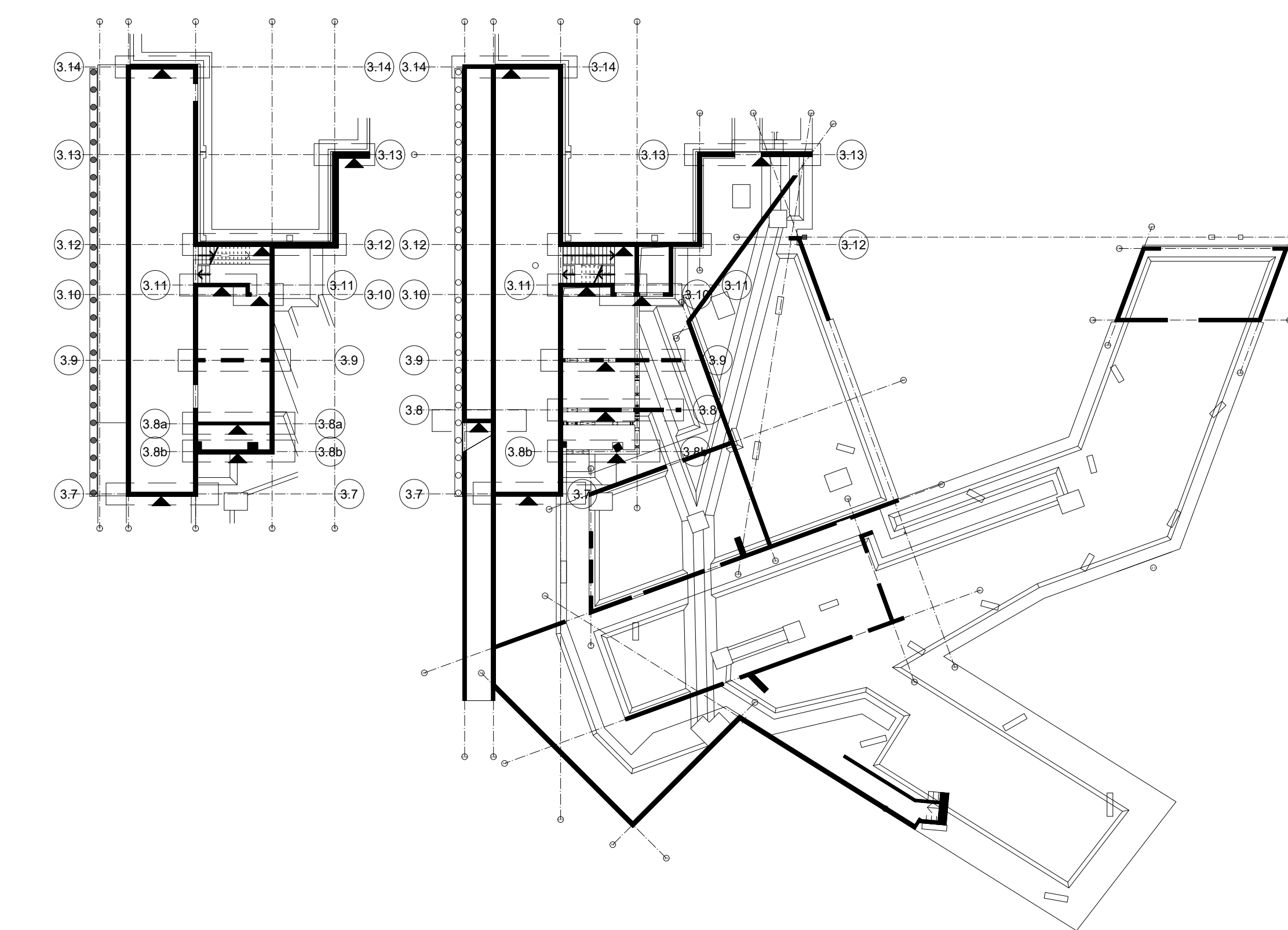
PREGLEDNI NACRT M 1:300
