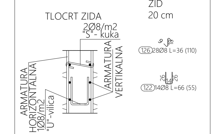
DETALJ POSTAVLJANJA DISTANCERA U ZID E-3
