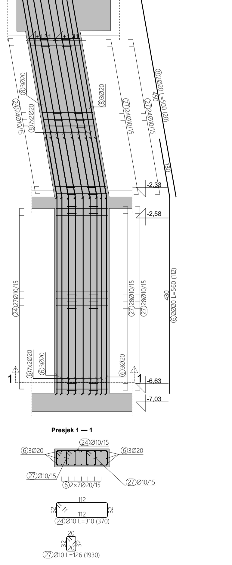
ARMATURA STUPA 3.9, M 1:50
