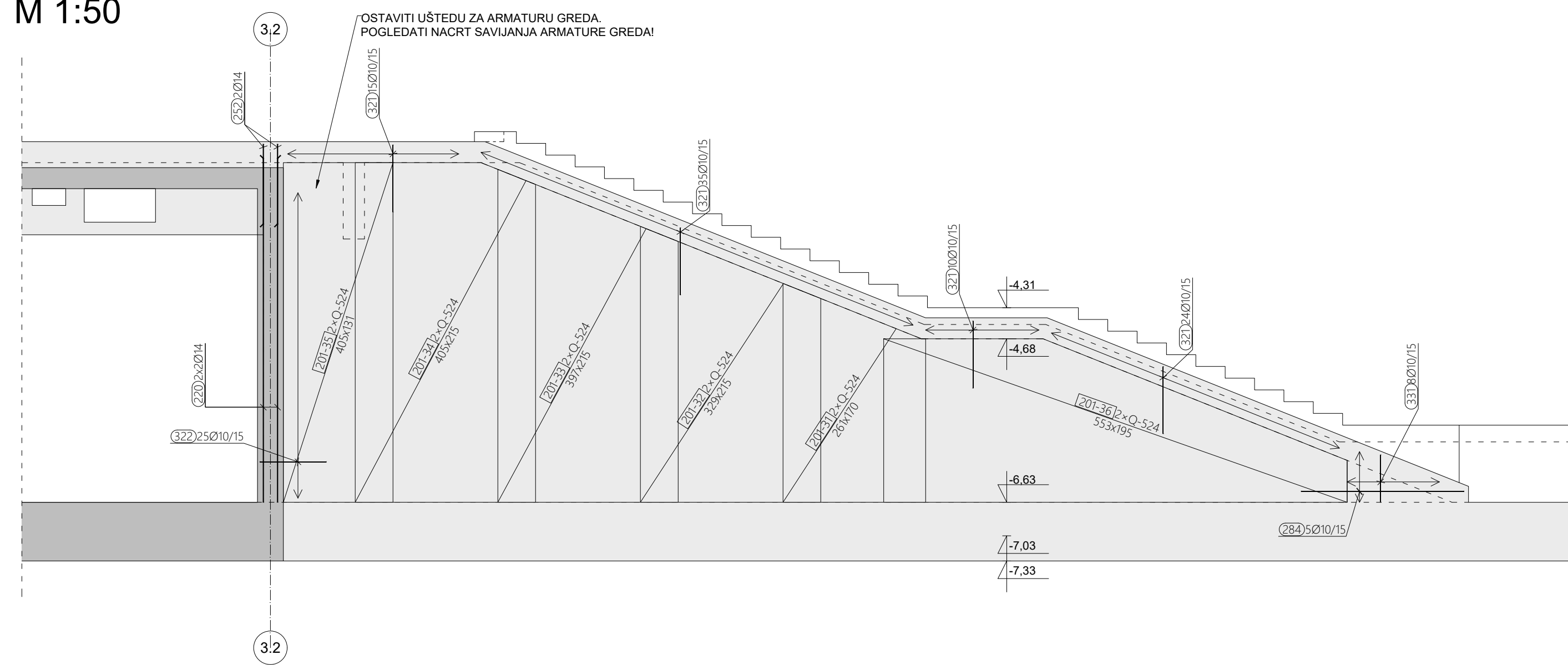
ARMATURA ZIDA U OSI 3.1, M 1:50
