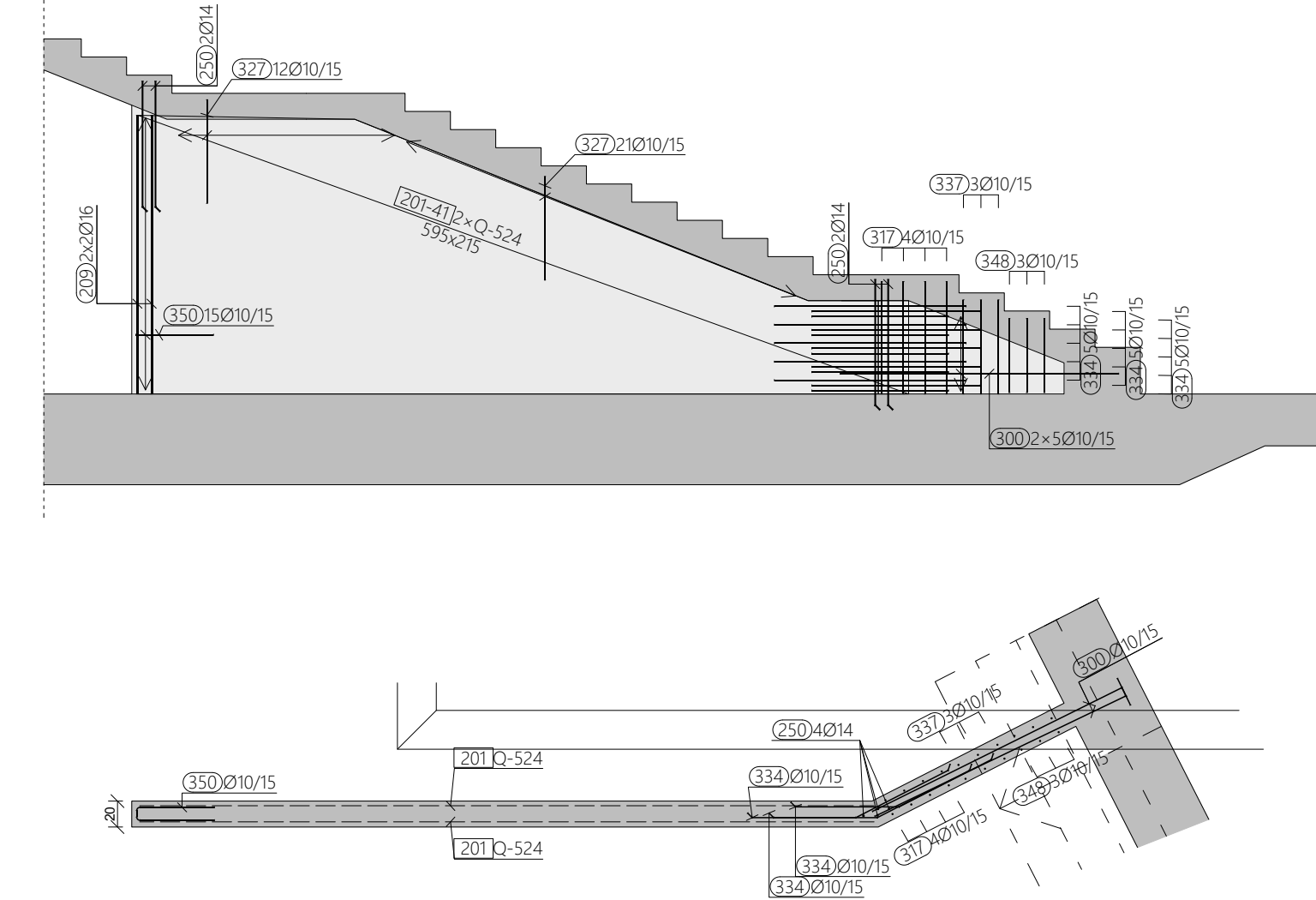
ARMATURA ZIDA KOD OSI 3.1, M 1:50
