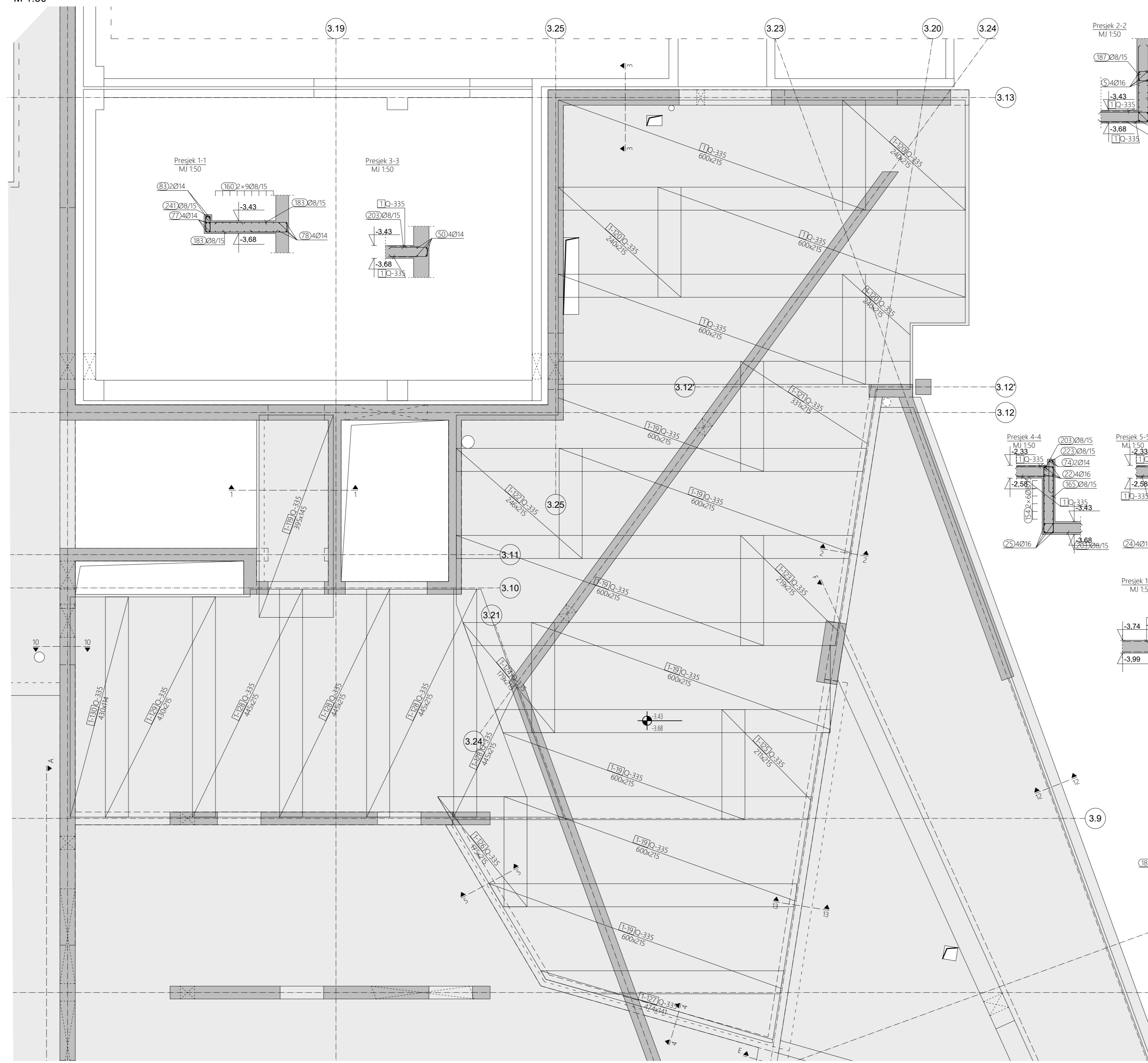
ARMATURA GORNJE ZONE, PLOČA NA VISINSKOJ KOTI -4.27/-4.52, M 1:50
