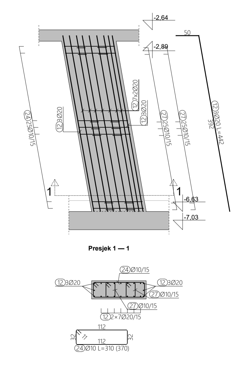
ARMATURA STUPA 3.15, (7 KOMADA) M 1:50
