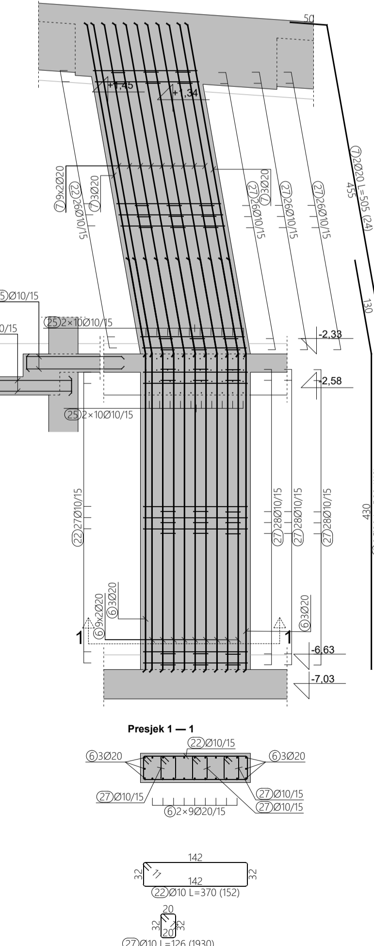
ARMATURA STUPA 3.11, M 1:50
