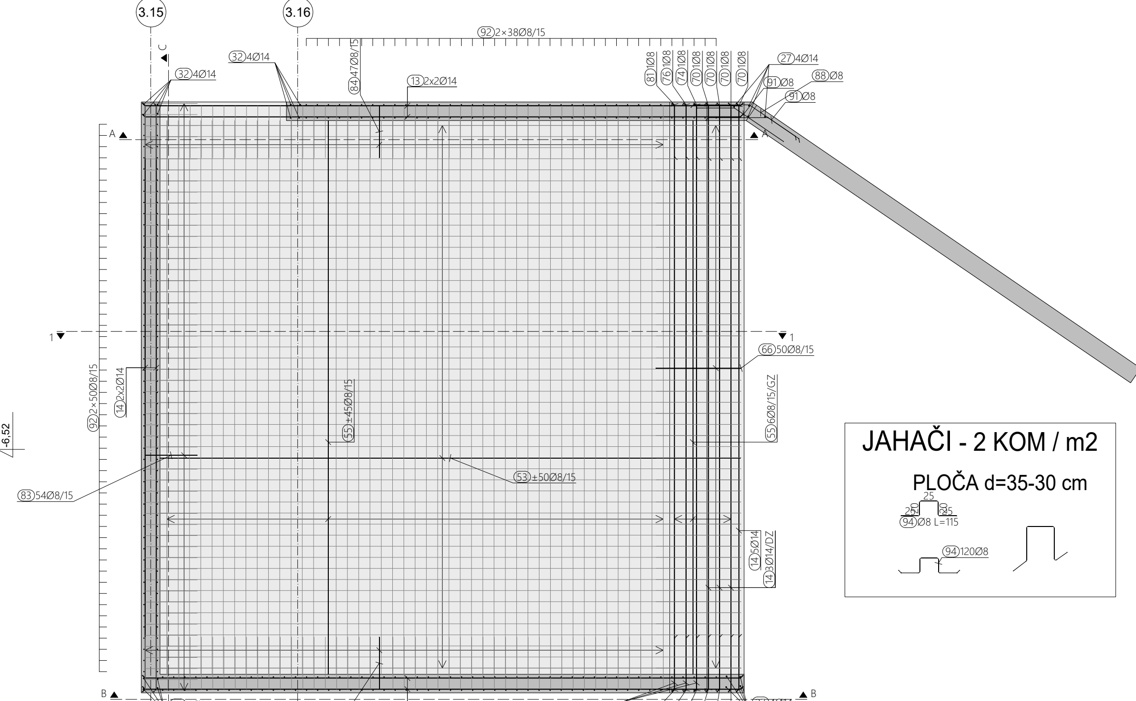
DONJA ZONA, RUBNA ARMATURA, ANKERI, GORNJA ZONA, M 1:50
