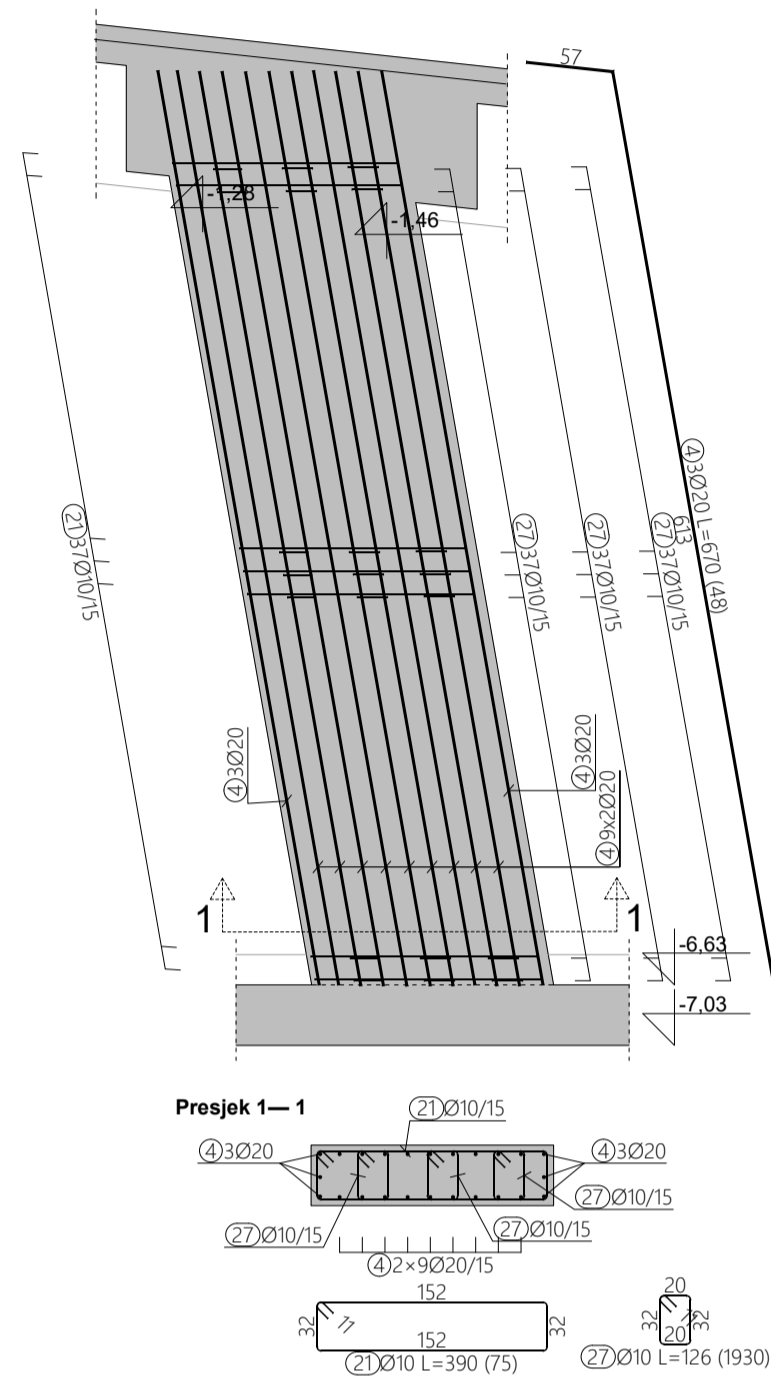
ARMATURA STUPA 3.8, M 1:50
