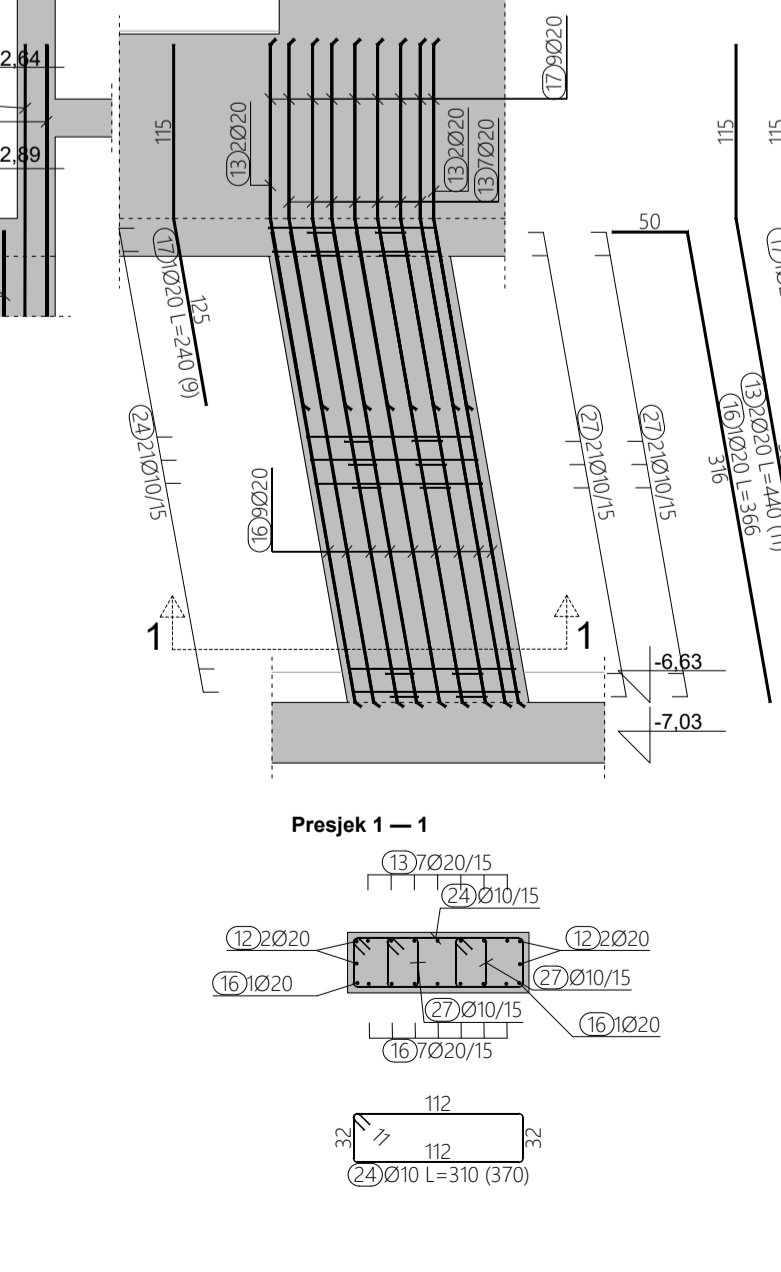
ARMATURA STUPA 3.14, M 1:50
