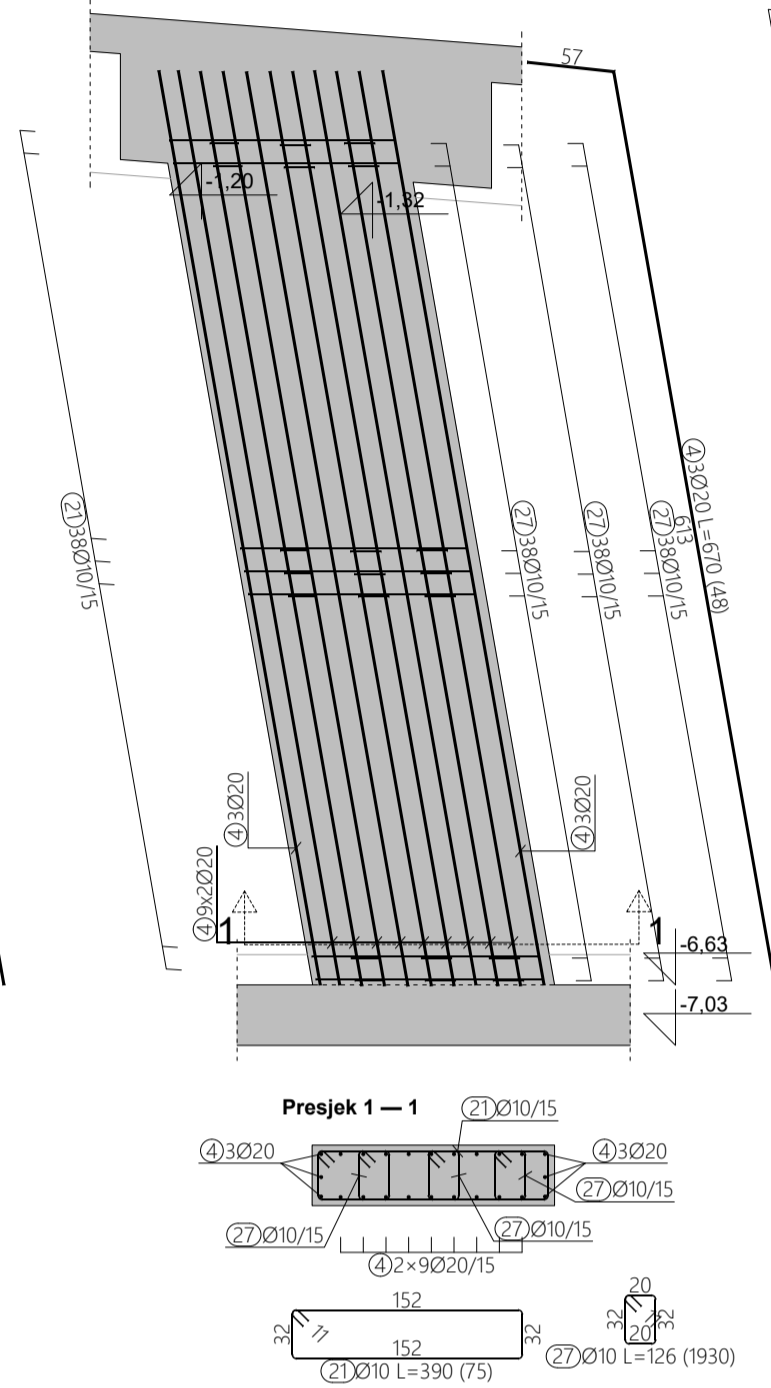
ARMATURA STUPA 3.9, M 1:50
