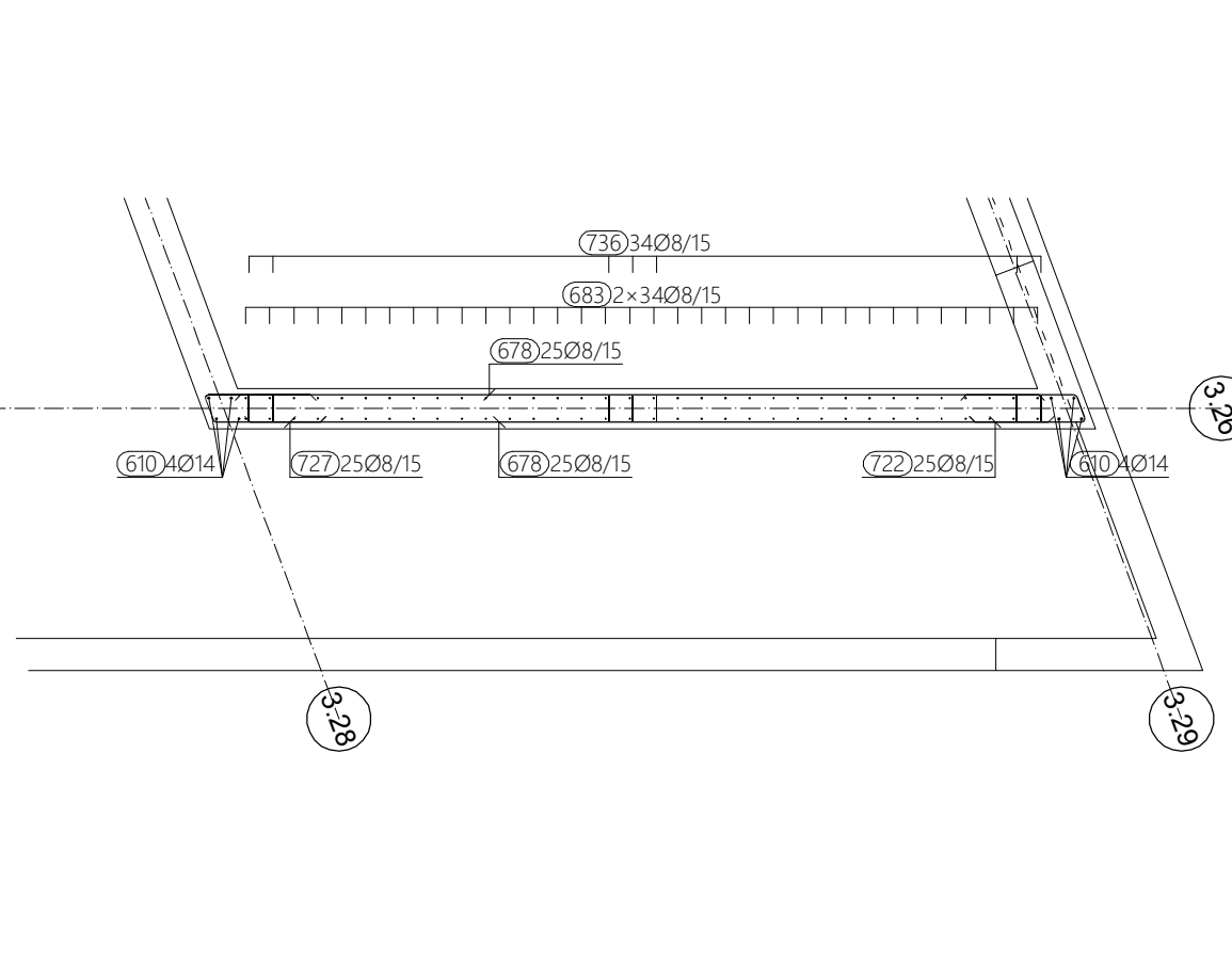
ARMATURA ZIDA U OSI 3.26 M 1:50
