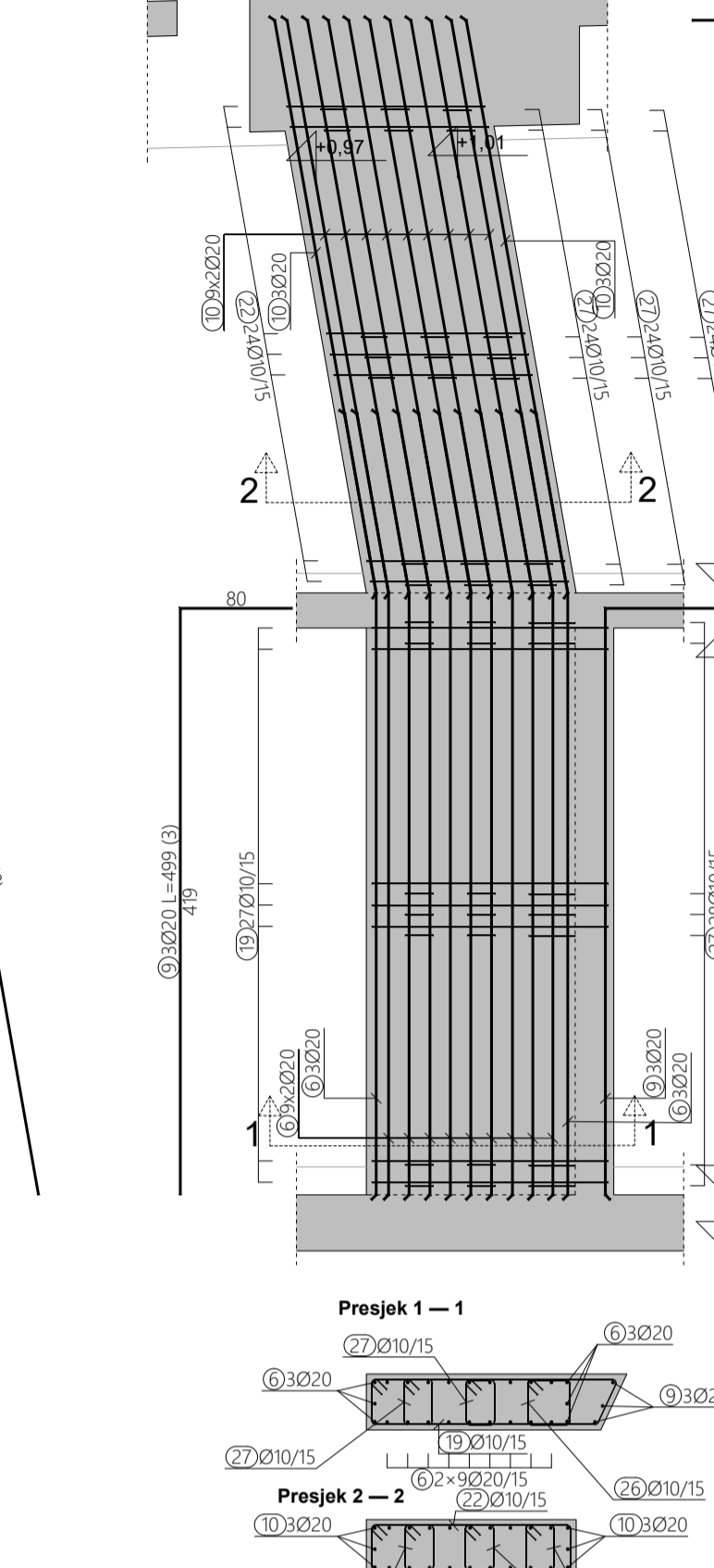
ARMATURA STUPA 3.7, M 1:50
