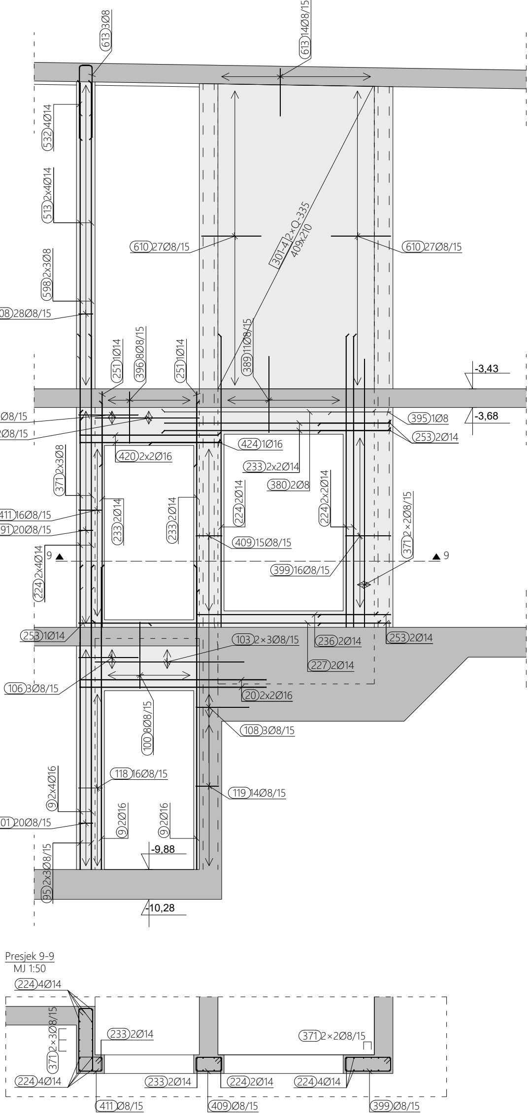
ARMATURA ZIDA U OSI 3.10, M 1:50
