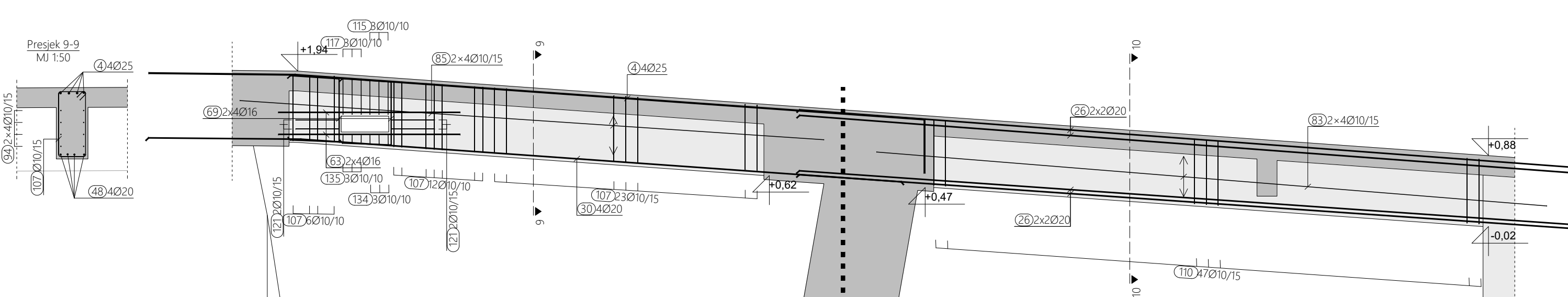
ARMATURA GREDE 3.19, M 1:50
