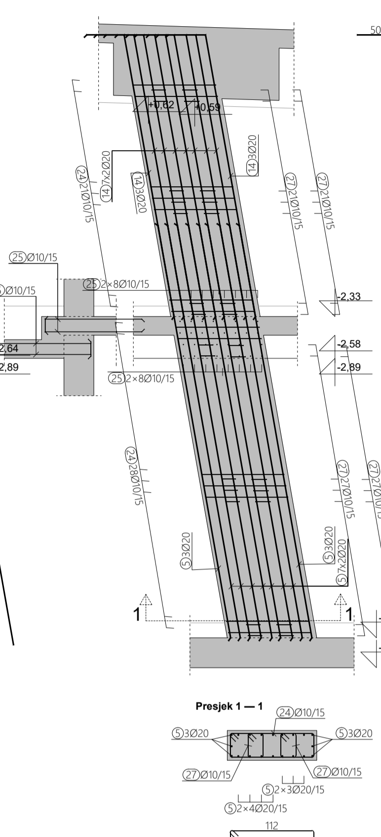
ARMATURA STUPA 3.6, M 1:50
