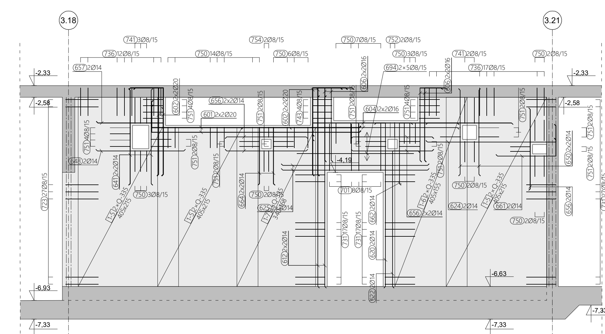
ARMATURA ZIDA U OSI 3.6 M 1:50
