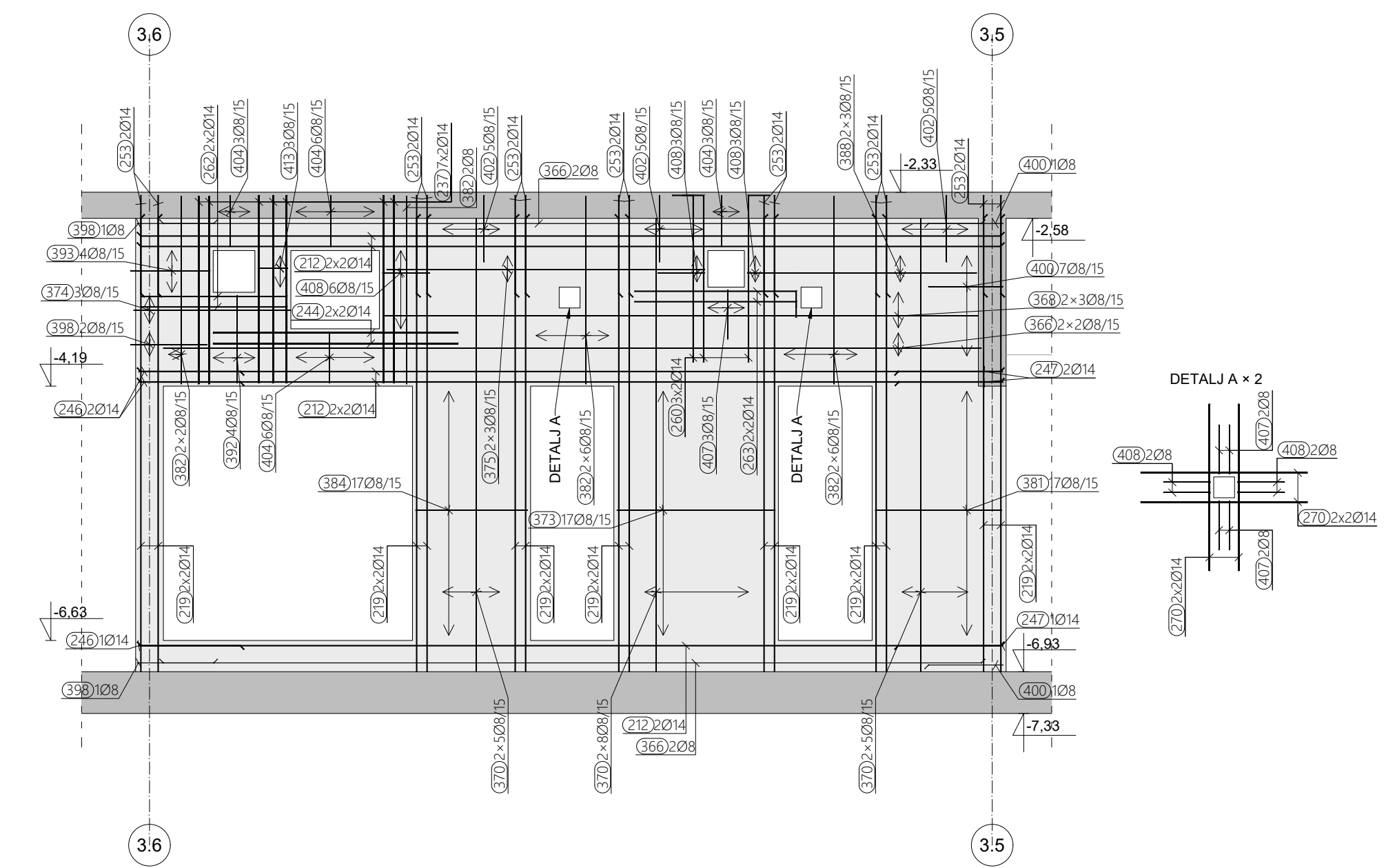
ARMATURA ZIDA U OSI 3.18, M 1:50
