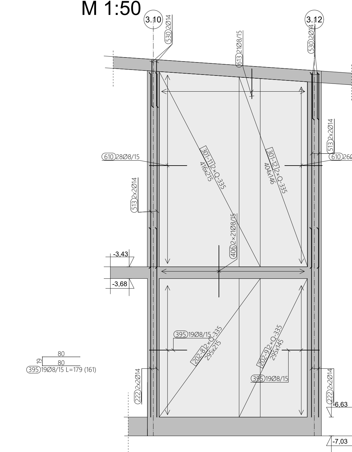
ARMATURA ZIDA KOD OSI 3.19 (ZID LIFTA), M 1:50
