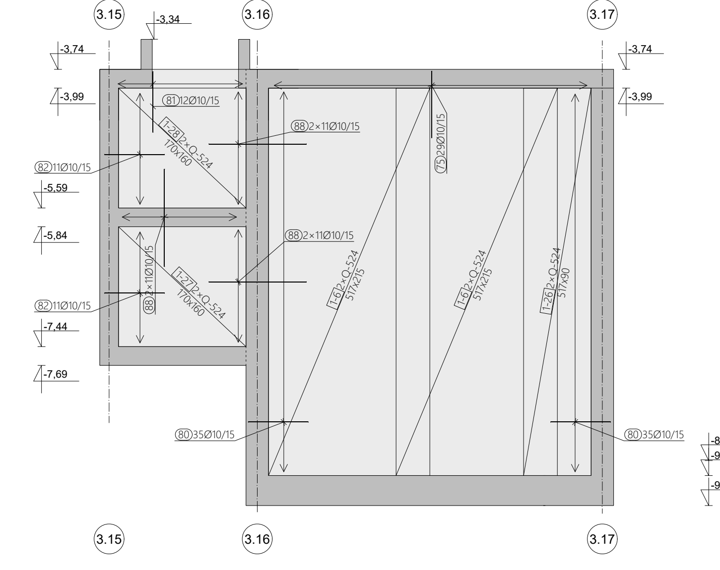
ARMATURA ZIDA U OSI 3.14, M 1:50
