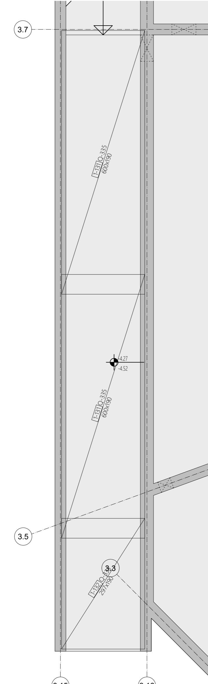
ARMATURA GORNJE ZONE, PLOČA NA VISINSKOJ KOTI -4.27/-4.52, M 1:50
