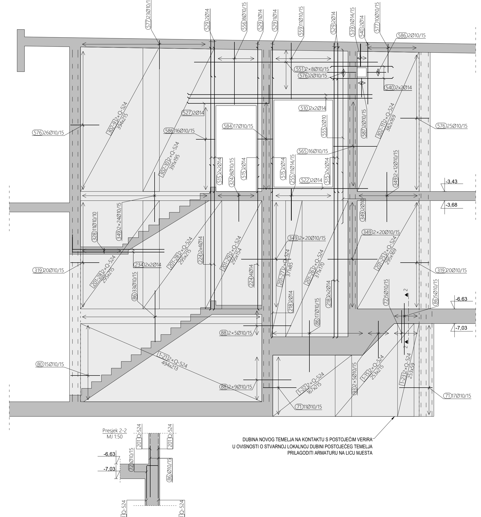
ARMATURA ZIDA U OSI 3.12, M 1:50
