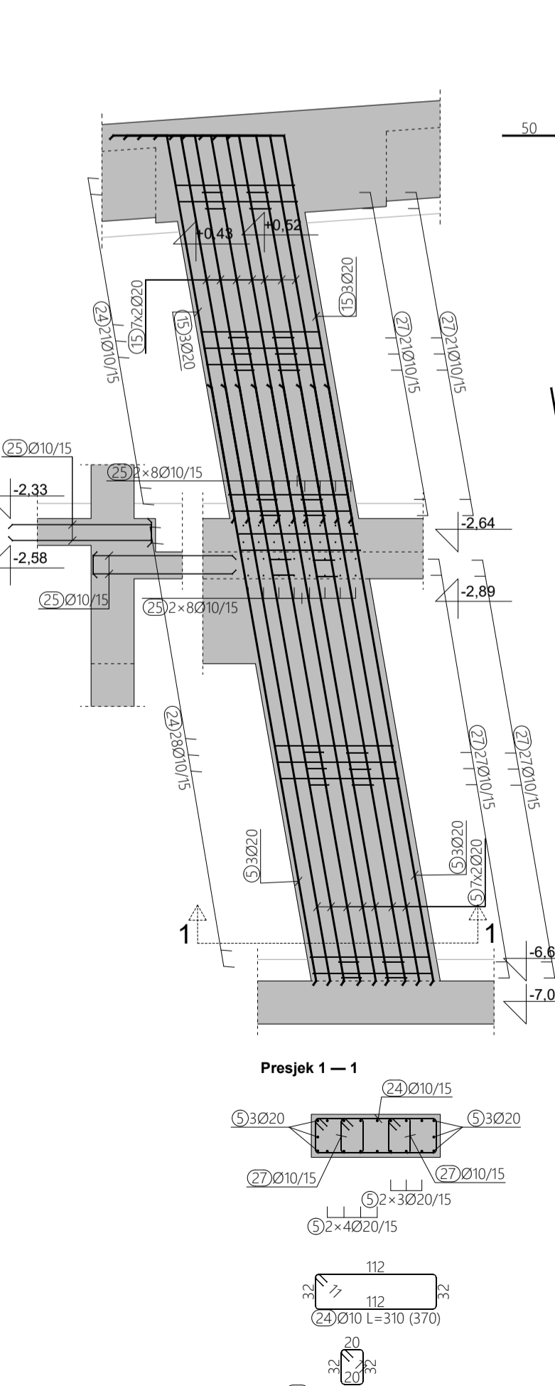
ARMATURA STUPA 3.12, M 1:50
