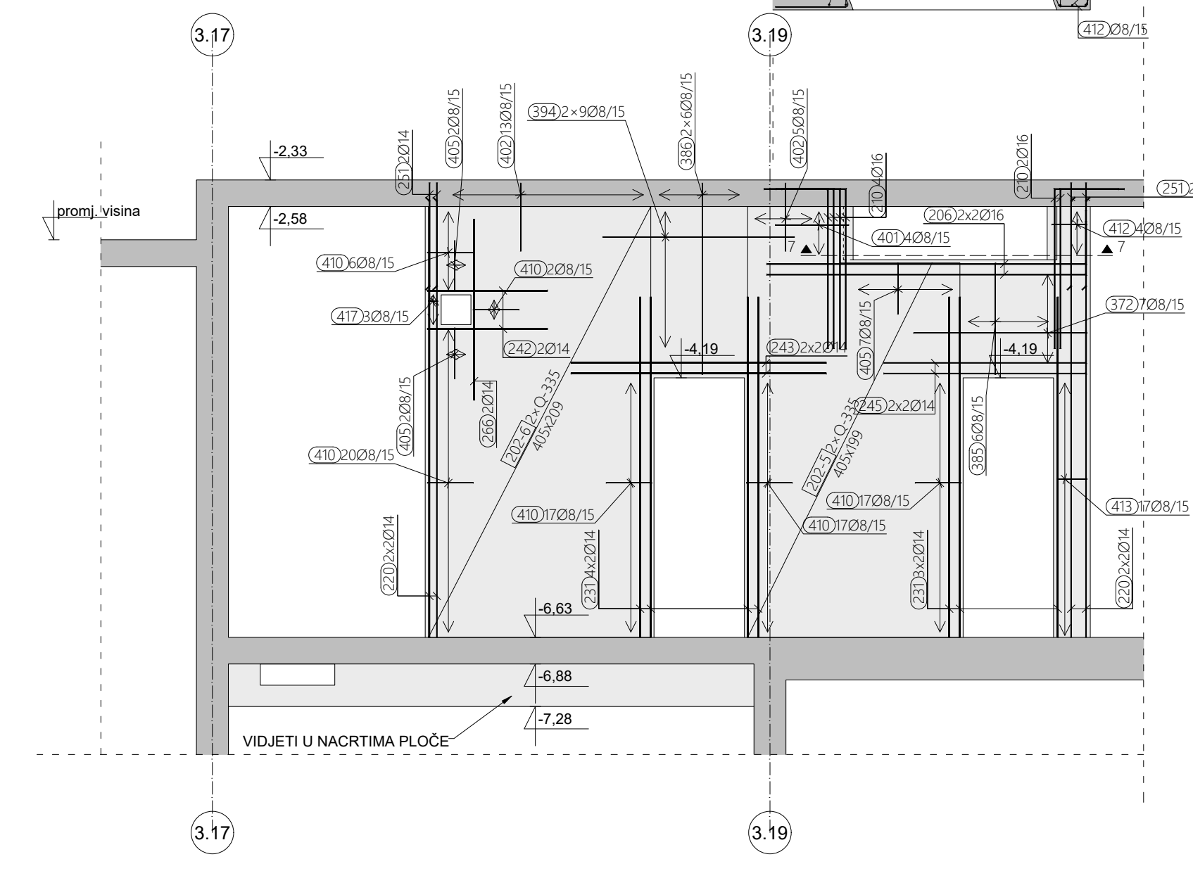
ARMATURA ZIDA U OSI 3.8, M 1:50
