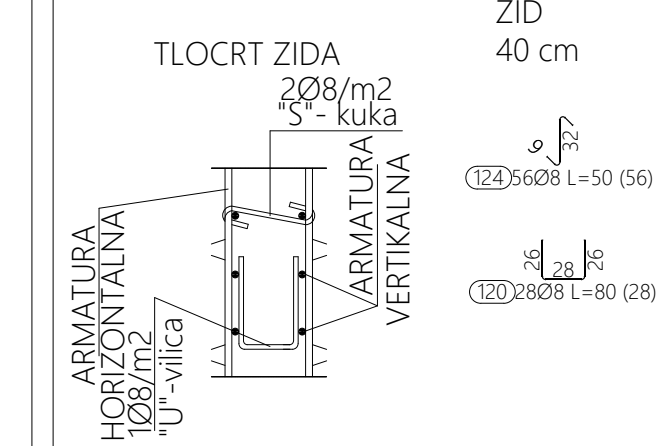
DETALJ POSTAVLJANJA DISTANCERA U ZID E-3
