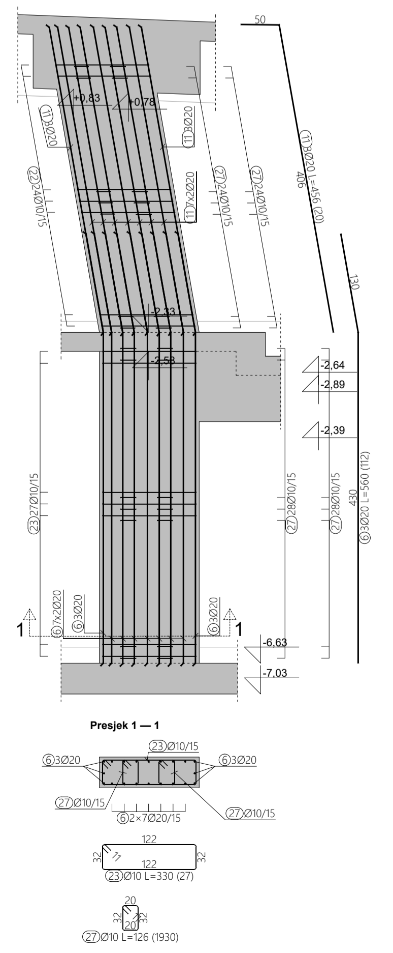
ARMATURA STUPA 3.8, M 1:50
