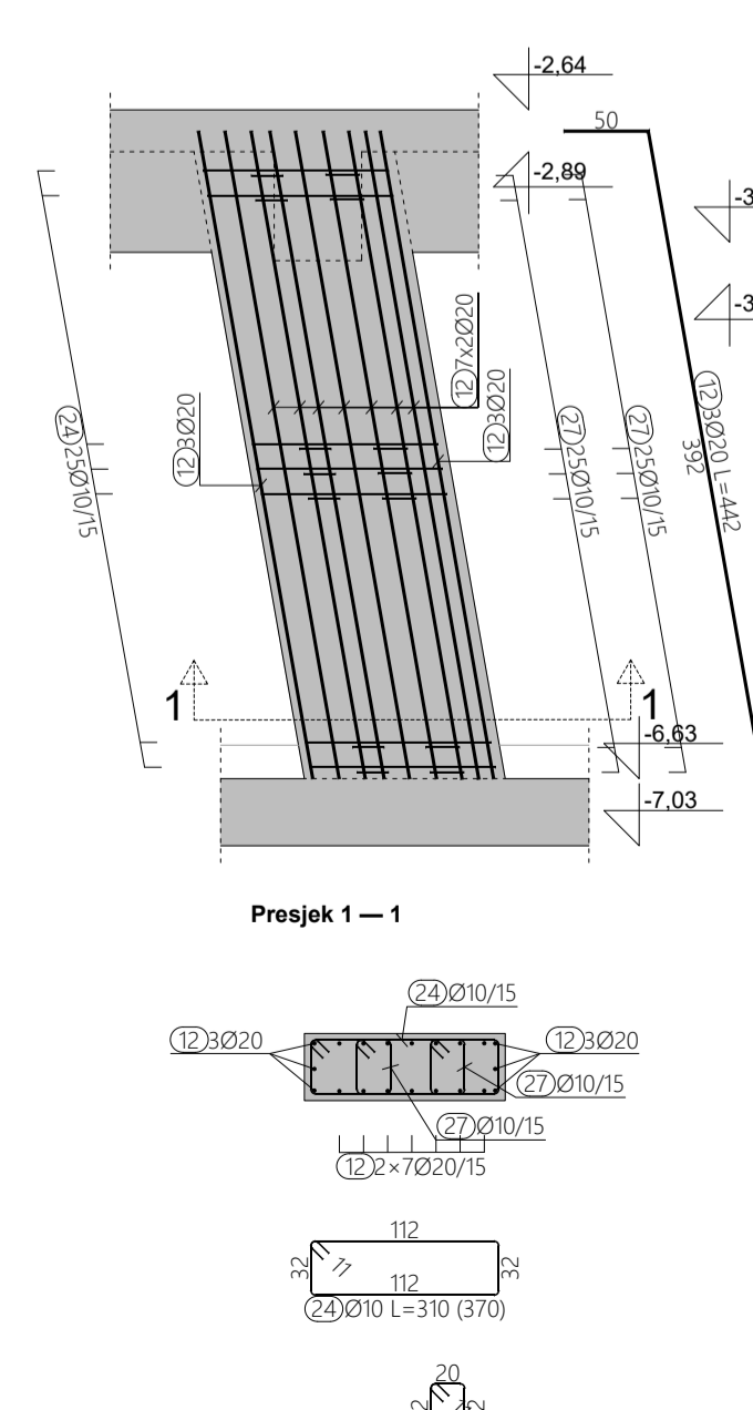
ARMATURA STUPA 3.13, M 1:50
