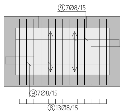
POGLED NA ZID U OSI 1
