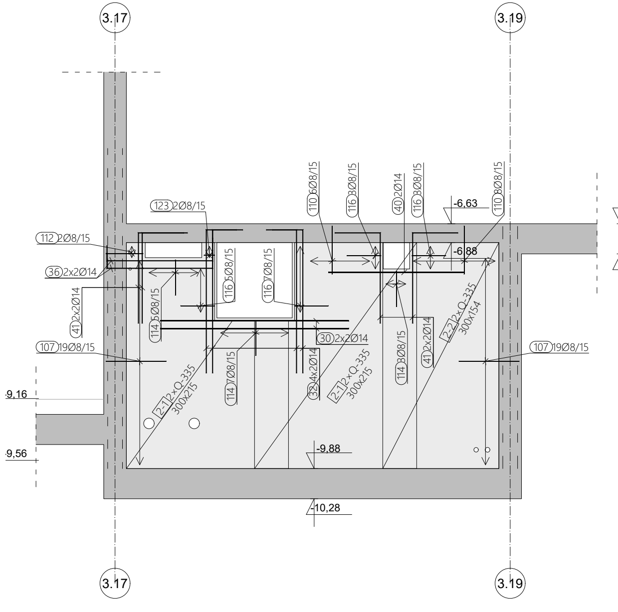
ARMATURA ZIDA U OSI 3.8a, M 1:50
