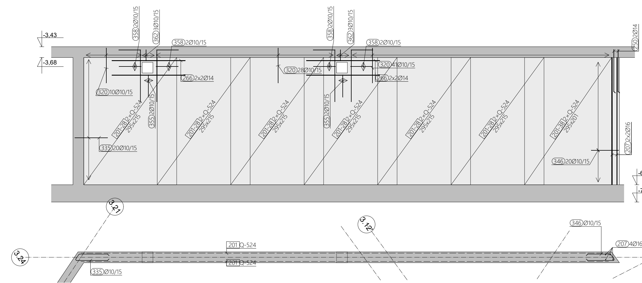
ARMATURA ZIDA U OSI 3.24, M 1:50
