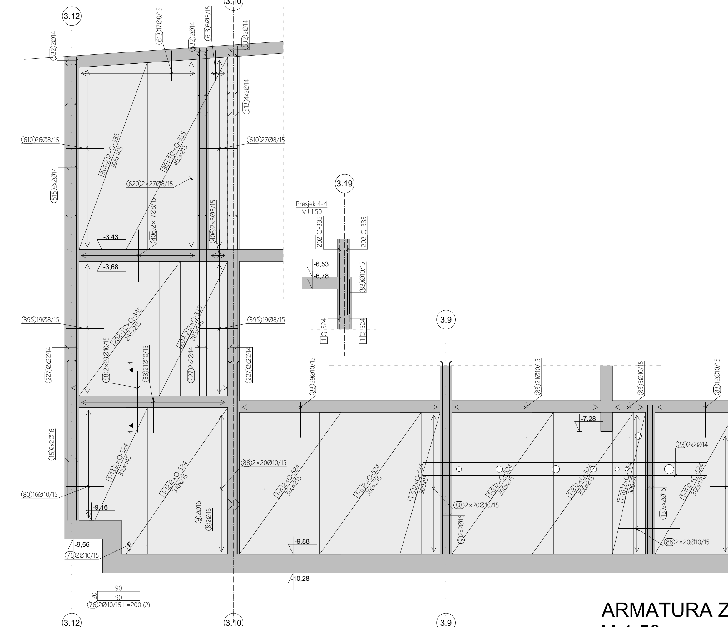
ARMATURA ZIDA U OSI 3.19, M 1:50
