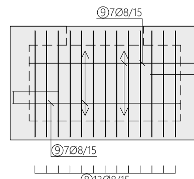
POGLED NA ZID U OSI 2
