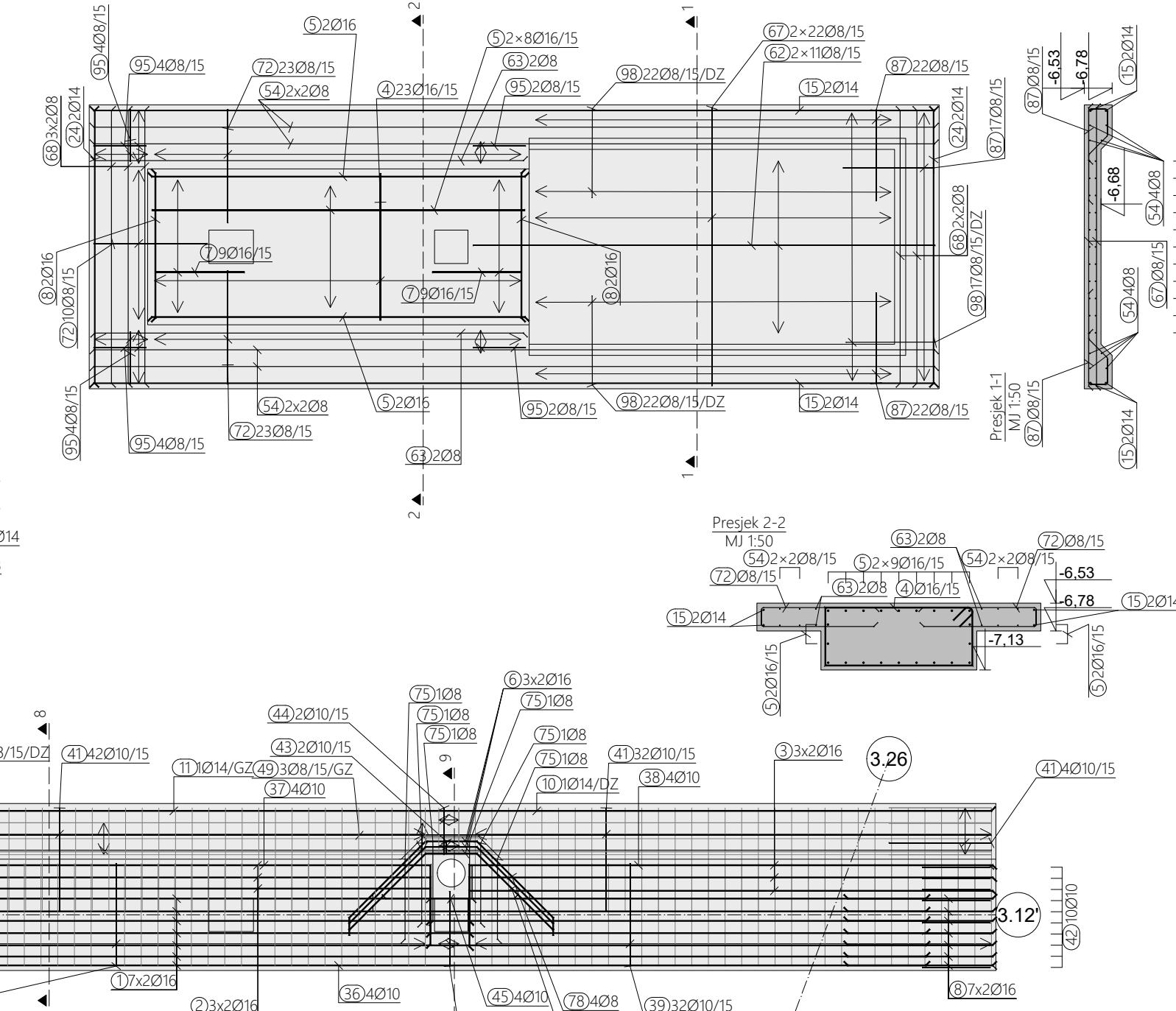
DONJA ZONA, RUBNA ARMATURA, ANKERI, GORNJA ZONA, M 1:50
