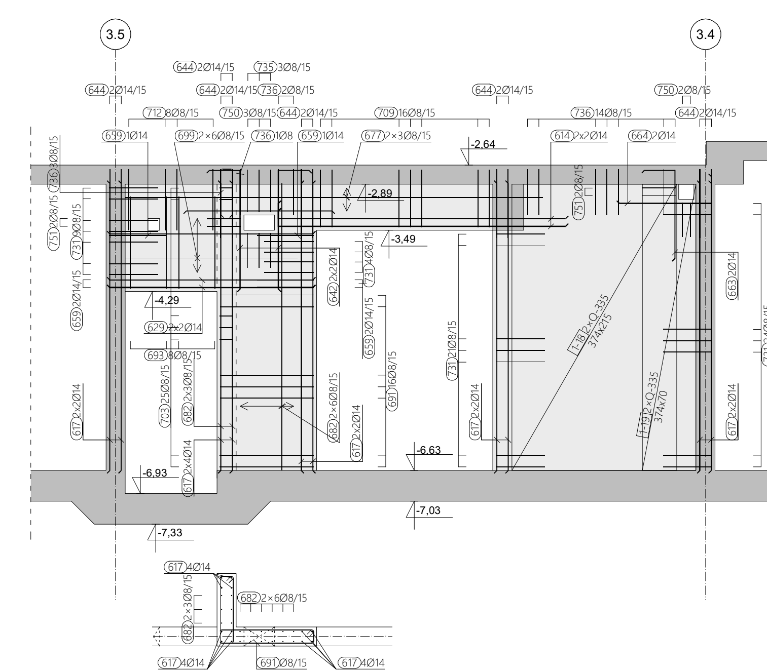
ARMATURA ZIDA U OSI 3.22 M 1:50
