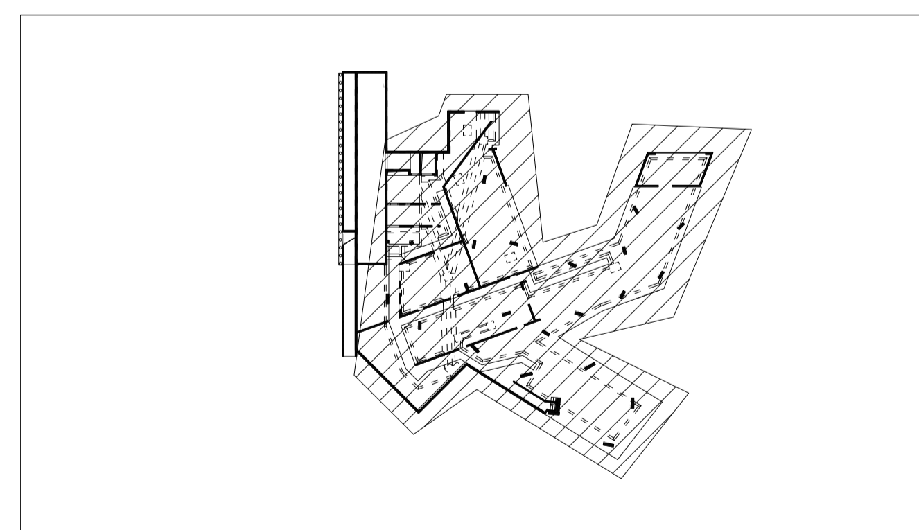
ARMATURA STUPA 3.15, (7 KOMADA) M 1:50
