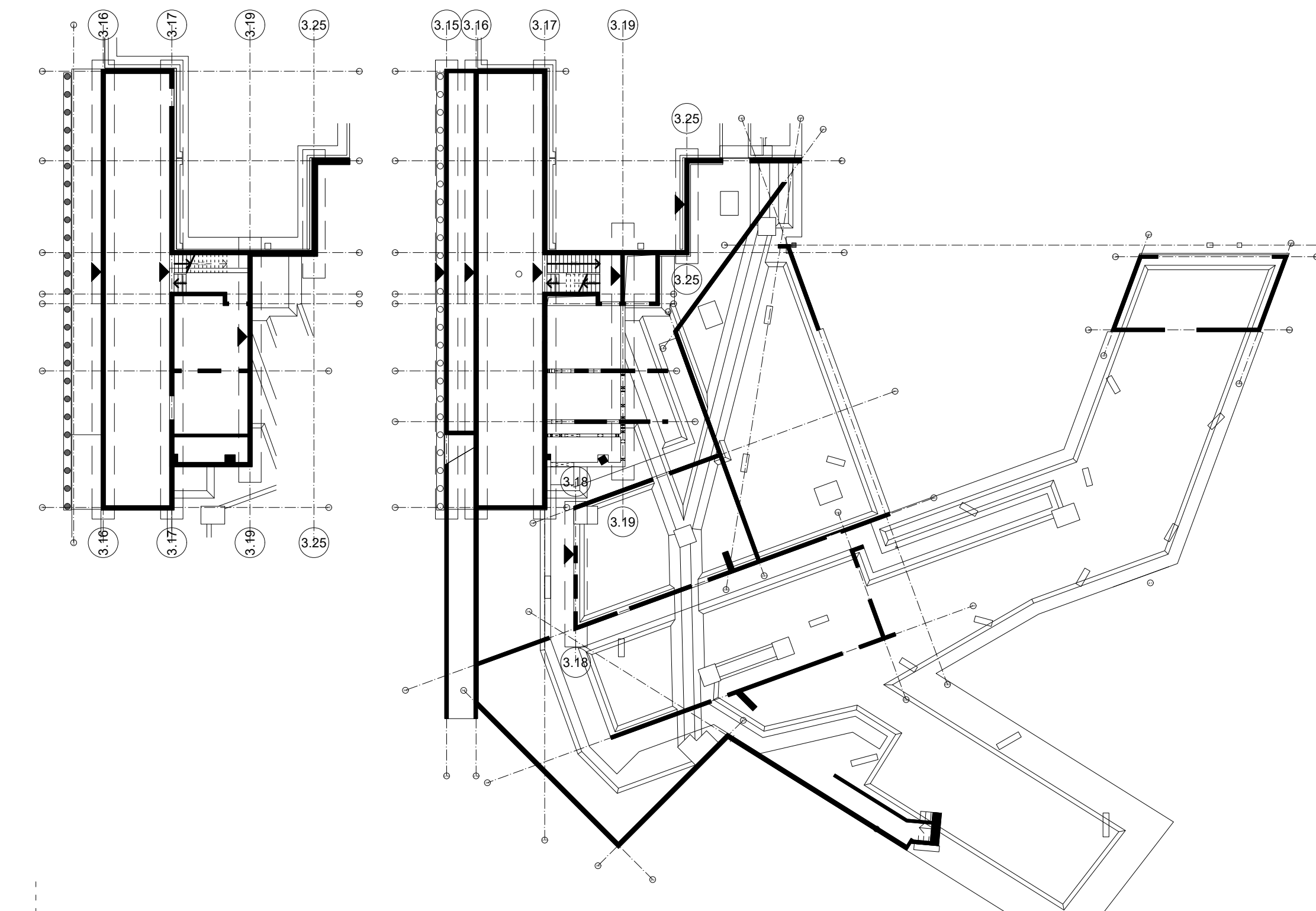
PREGLEDNI NACRT M 1:300
