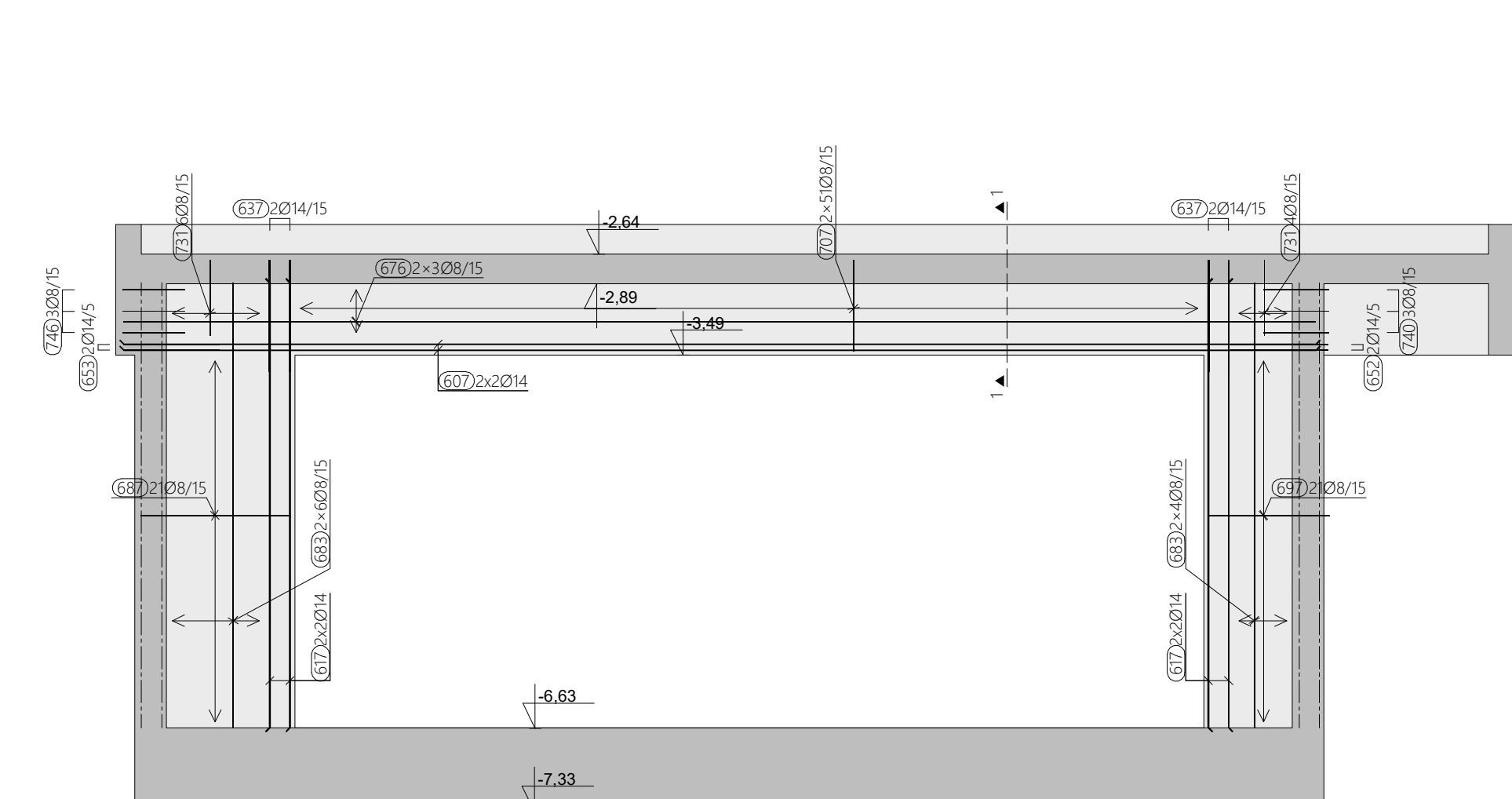
ARMATURA ZIDA U OSI 3.29 M 1:50
