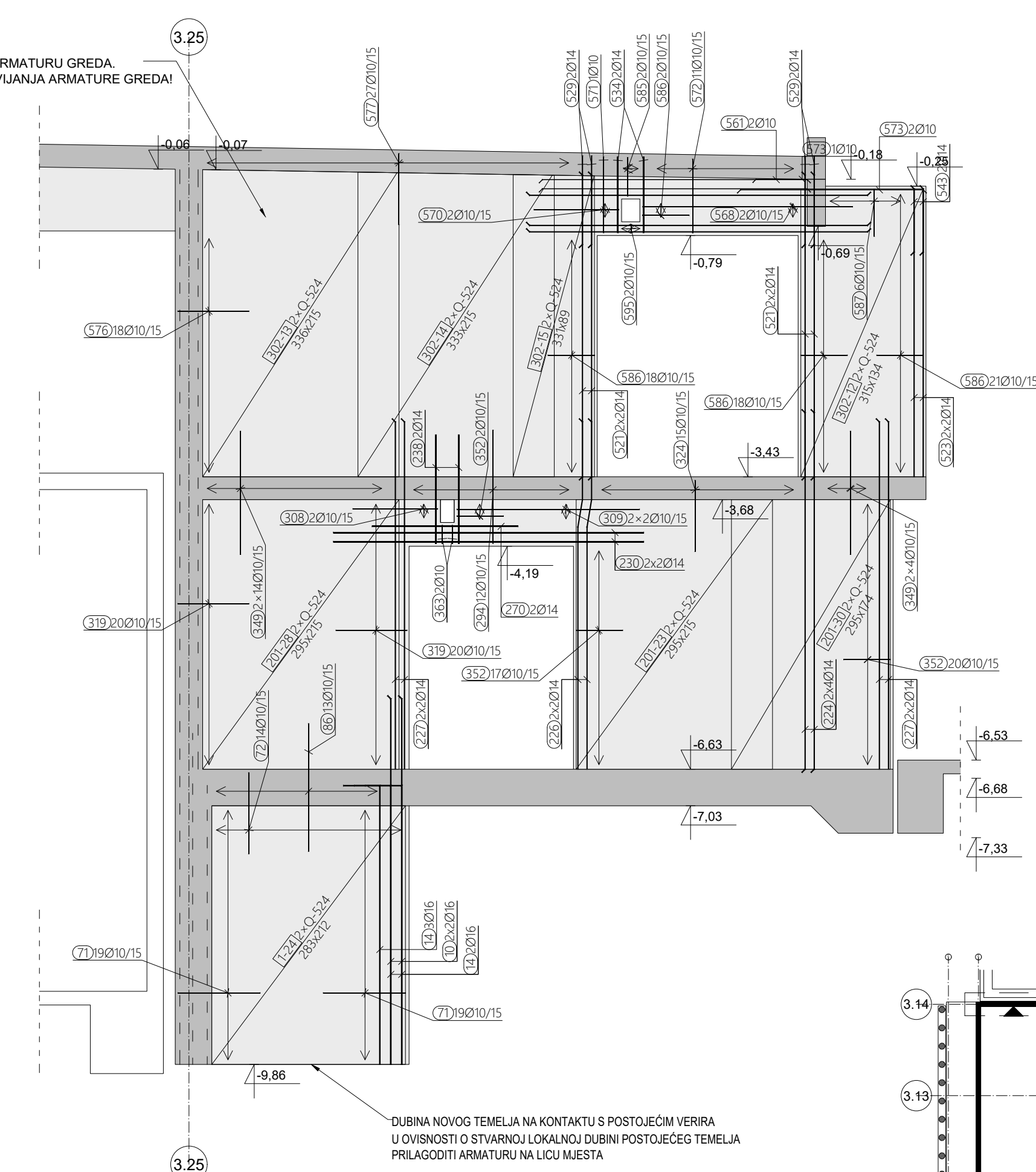
ARMATURA ZIDA U OSI 3.13, M 1:50
