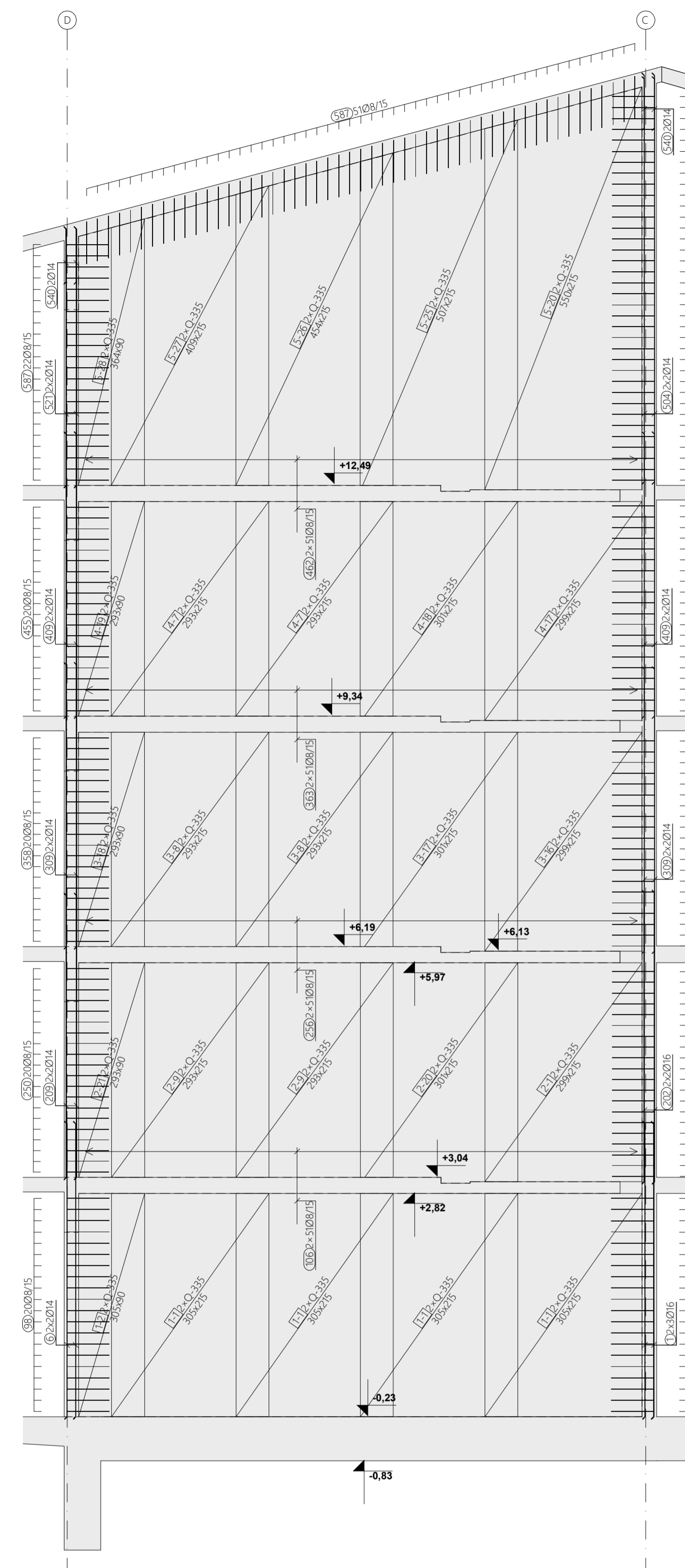
DETALJI POSTAVLJANJA DISTANCERA U ZIDOVE PRIZESTERA
