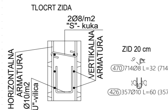
DETALJ POSTAVLJANJA DISTANCERA U ZIDOVE DRUGOG KATA
