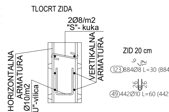
DETALJ POSTAVLJANJA DISTANCERA U ZIDOVE SUTERENA
