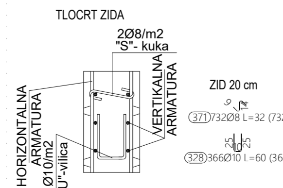
DETALJ POSTAVLJANJA DISTANCERA U ZIDOVE PRVOG KATA
