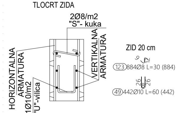
DETALJ POSTAVLJANJA DISTANCERA U ZIDOVE SUTERENA
