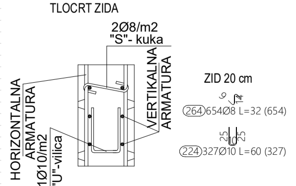
DETALJ POSTAVLJANJA DISTANCERA U ZIDOVE PRIZEMLJA
