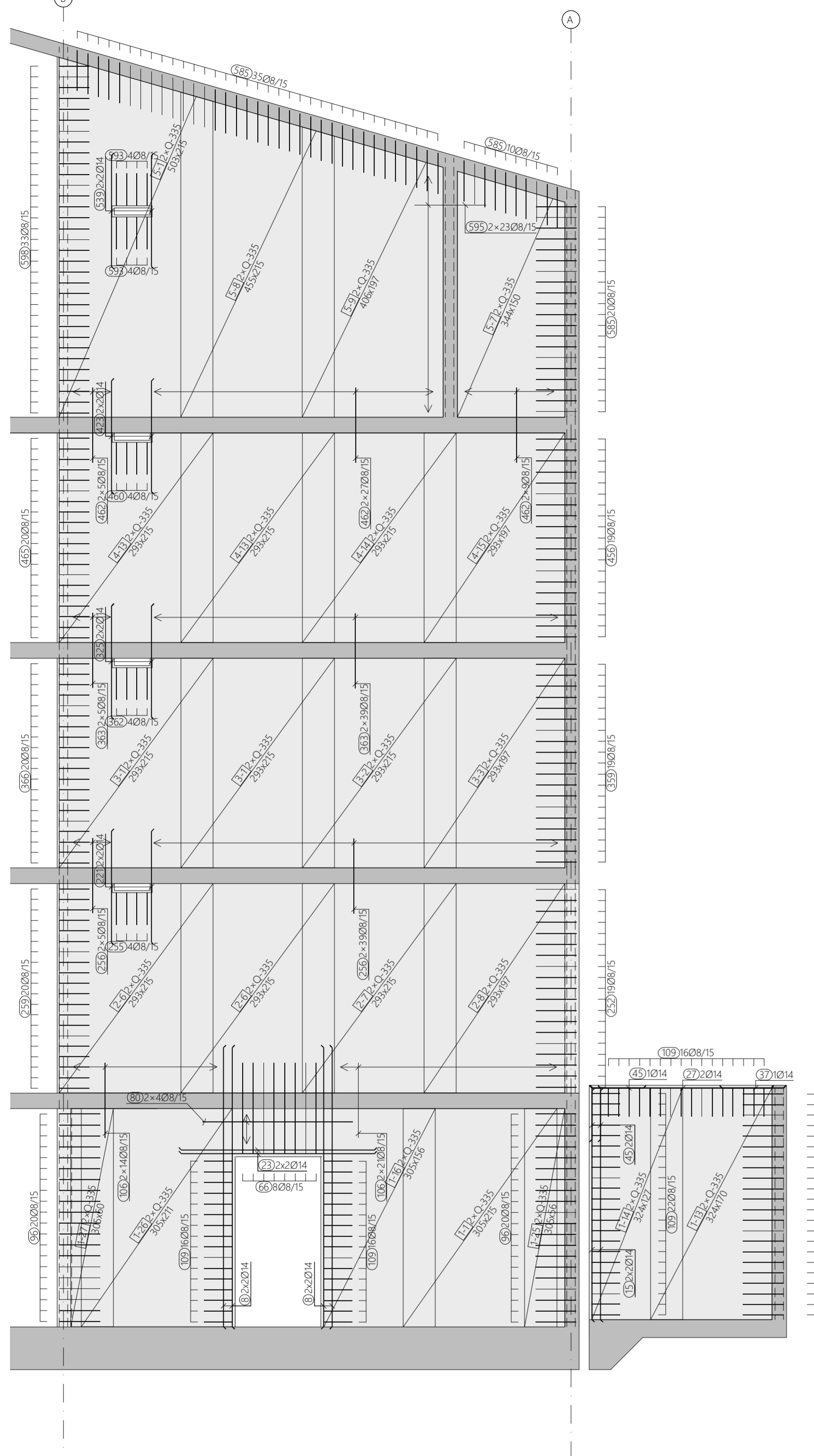
POGLED NA KOSI ZID U OSI 3
