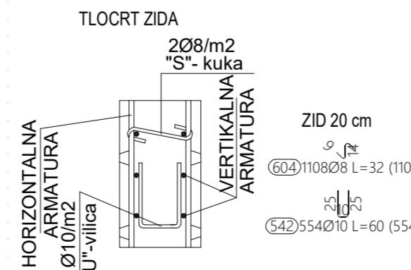
DETALJ POSTAVLJANJA DISTANCERA U ZIDOVE TREĆEG KATA
