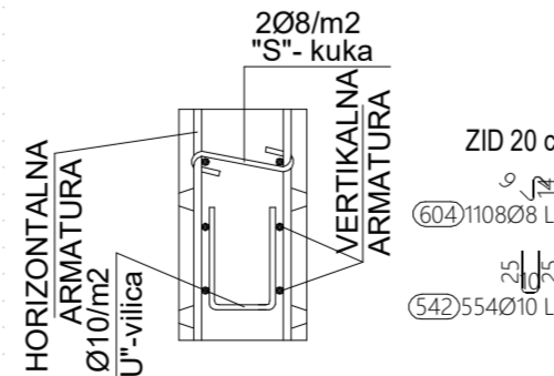
DETALJI POSTAVLJANJA DISTANCERA U ZIDOVE TREĆEG KATA
