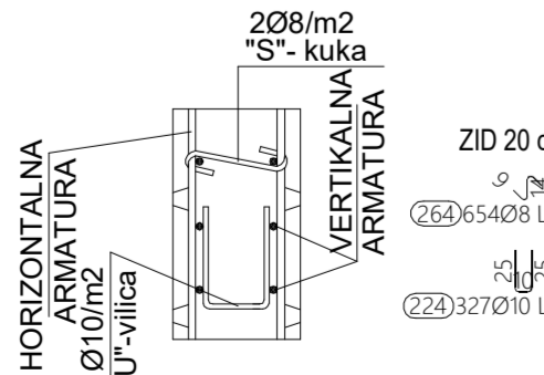
DETALJI POSTAVLJANJA DISTANCERA U ZIDOVE PRIZESTERA
