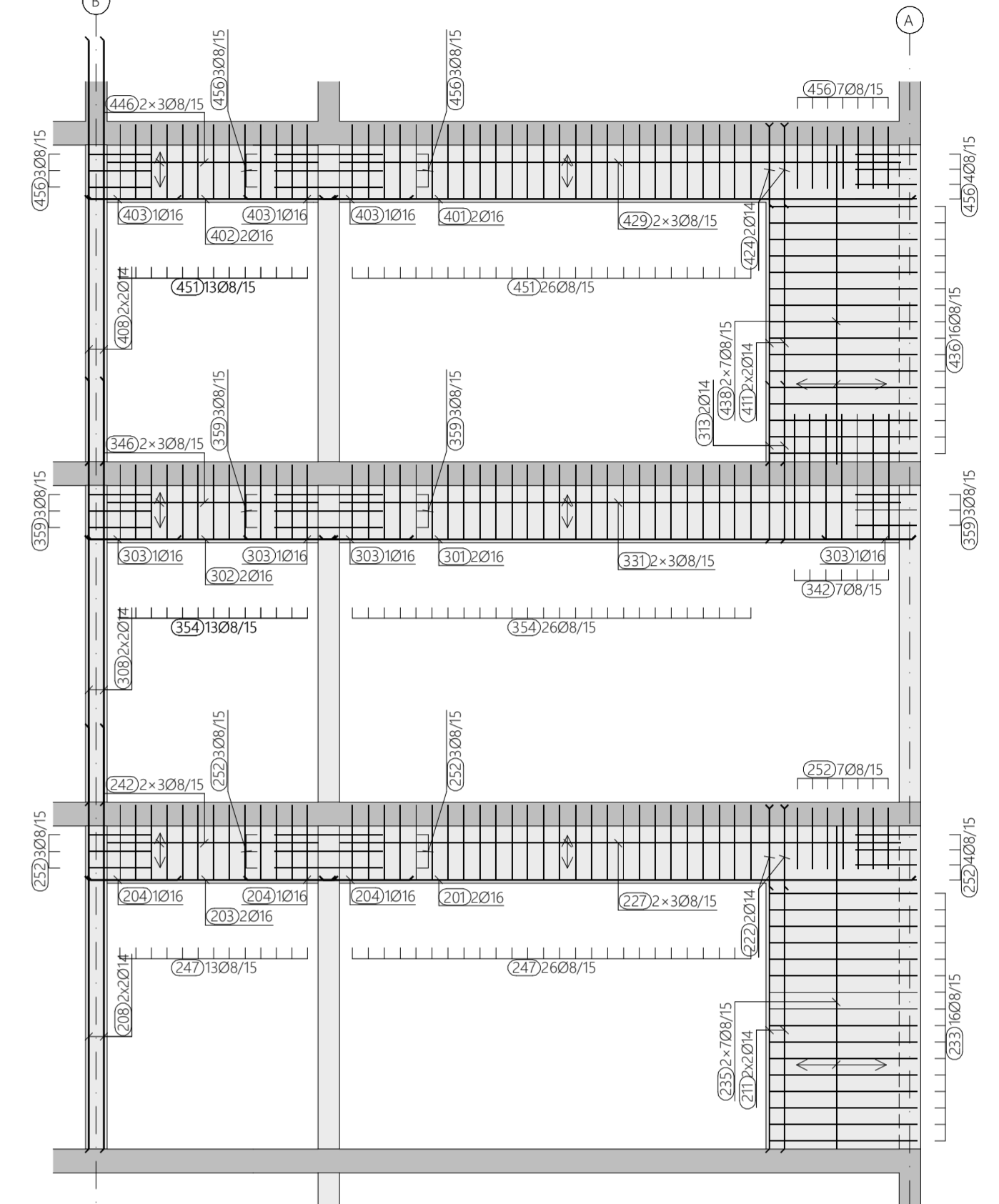
POGLED NA KOSI ZID U OSI 6
