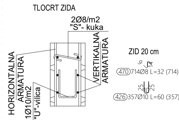
DETALJ POSTAVLJANJA DISTANCERA U ZIDOVE DRUGOG KATA
