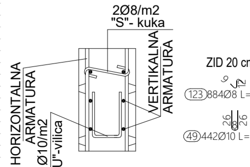
DETALJI POSTAVLJANJA DISTANCERA U ZIDOVE PRIZESTERA
