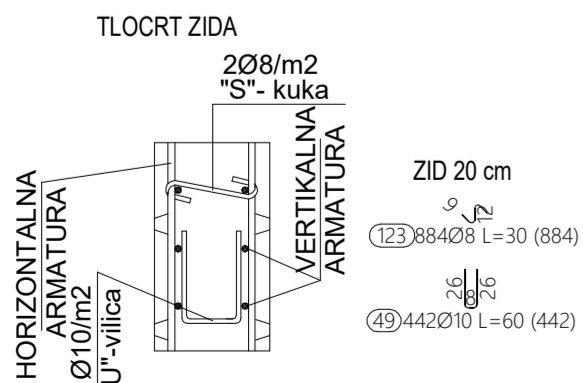
DETALJ POSTAVLJANJA DISTANCERA U ZIDOVE SUTERENA
