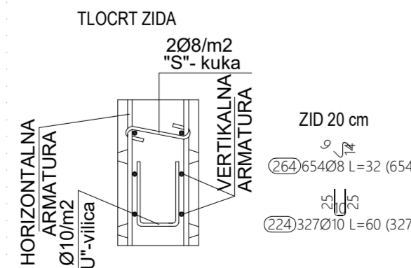
DETALJ POSTAVLJANJA DISTANCERA U ZIDOVE PRIZEMLJA
