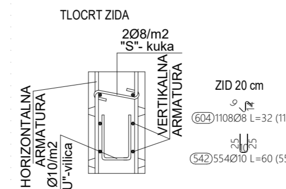
DETALJ POSTAVLJANJA DISTANCERA U ZIDOVE TREĆEG KATA
