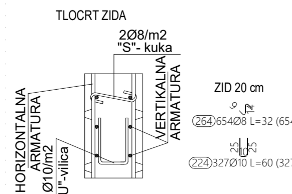
DETALJ POSTAVLJANJA DISTANCERA U ZIDOVE PRIZEMLJA
