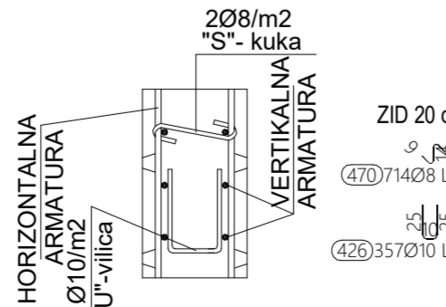
DETALJI POSTAVLJANJA DISTANCERA U ZIDOVE DRUGOG KATA
