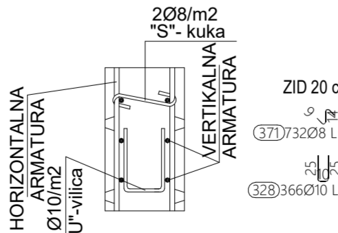
DETALJI POSTAVLJANJA DISTANCERA U ZIDOVE PRVOG KATA
