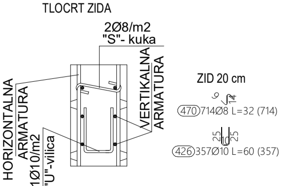
DETALJ POSTAVLJANJA DISTANCERA U ZIDOVE DRUGOG KATA
