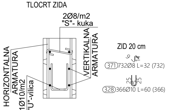
DETALJ POSTAVLJANJA DISTANCERA U ZIDOVE PRVOG KATA
