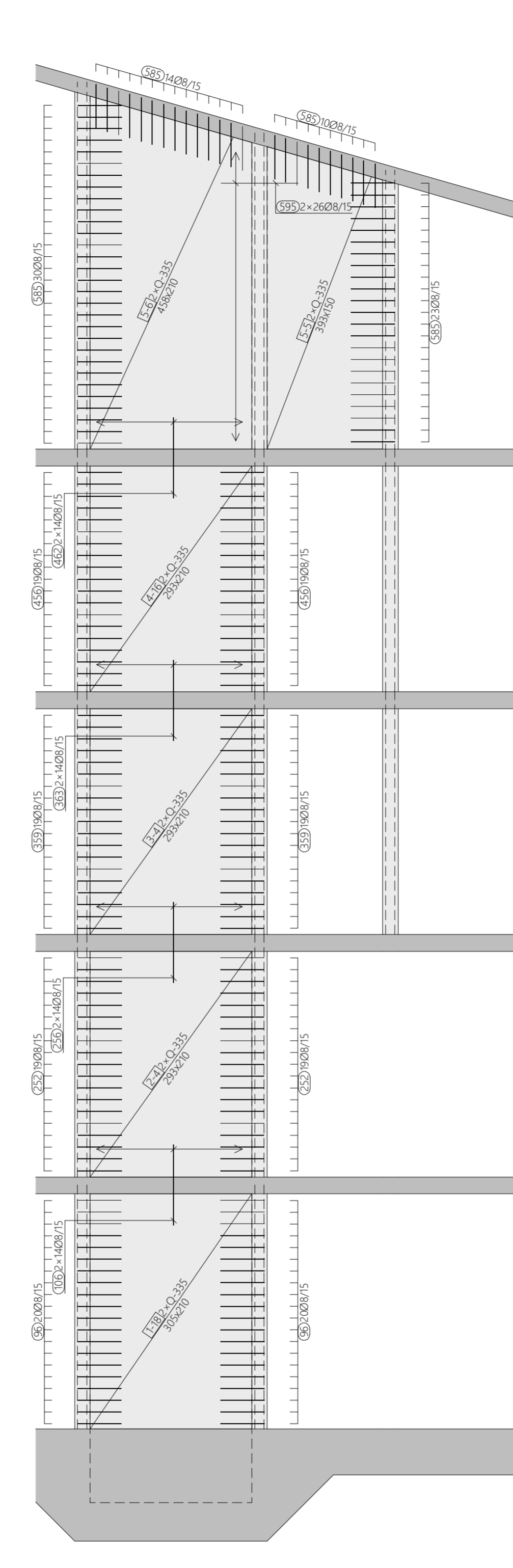
POGLED NA KOSI ZID IZMEĐU OSI 6 I 7
